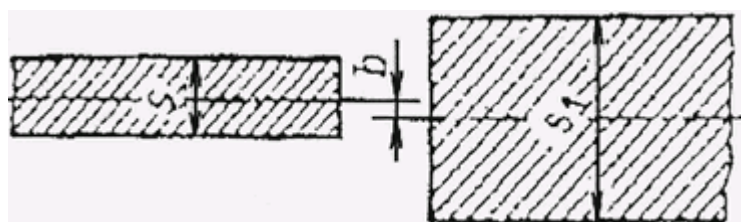
Рис.2. Смещение кромок листов (не приводится)
