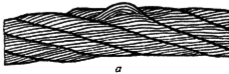
Рис.11. Выдавливание сердечника
