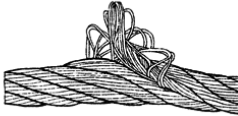
Рис.11. Выдавливание сердечника
