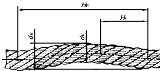
Рис.2. Волнистость каната
