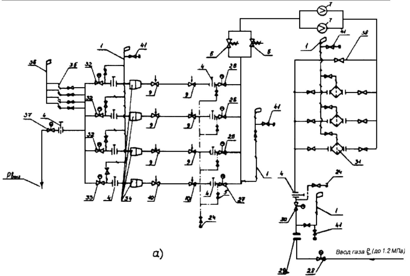
Рисунок Ж.1 - Типовая схема газопроводов
