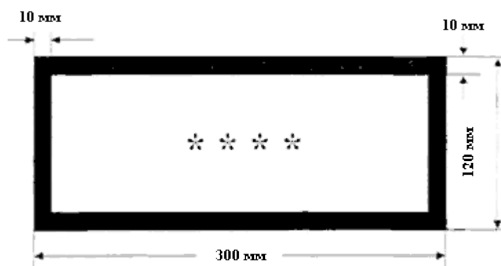
Рис.7. Предупредительный знак для отдельного изображения номера ООН. Цвет фона знака - оранжевый, рамка и номер ООН - черные. Знак **** обозначает место, где должен помещаться соответствующий номер ООН для радиоактивного материала согласно приложению 5
