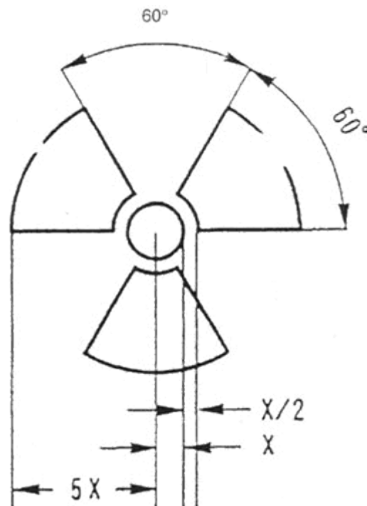
Рис.1. Основной знак радиационной опасности в виде трилистника, пропорции которого определяются по центральной окружности радиуса X . Минимальная допустимая величина X равна 4 мм
