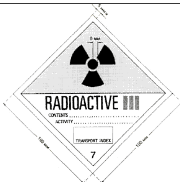
Рис.3. Этикетка категории III - ЖЕЛТАЯ (III - YELLOW). Цвет фона верхней половины этикетки - желтый, нижней половины - белый, цвет основного знака радиационной опасности (трилистника) и надписей - черный, цвет полос, обозначающих категорию, - красный
