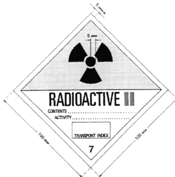
Рис.2. Этикетка категории II - ЖЕЛТАЯ (II - YELLOW). Цвет фона верхней половины этикетки - желтый, нижней половины - белый, цвет основного знака радиационной опасности (трилистника) и надписей - черный, цвет полос, обозначающих категорию, - красный
