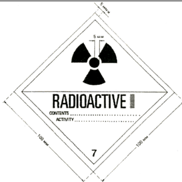
Рис.1. Этикетка категории I - БЕЛАЯ (I - WHITE). Цвет фона этикетки - белый, цвет основного знака радиационной опасности (трилистника) и надписей - черный, цвет полосы, обозначающей категорию, - красный
