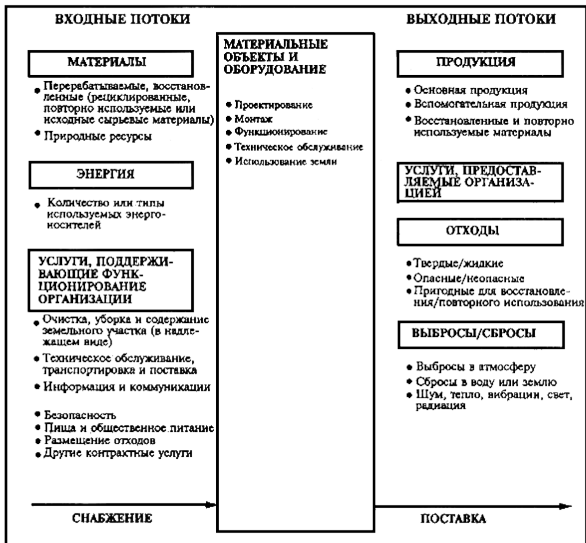
Рисунок А.1 - Схема функционирования организации (с дополнительными деталями) А.4.3.2 Примеры ПЭФ
