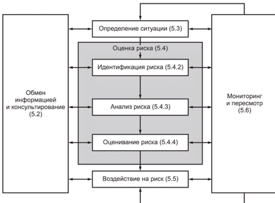
Рисунок 3 - Процесс риск-менеджмента
