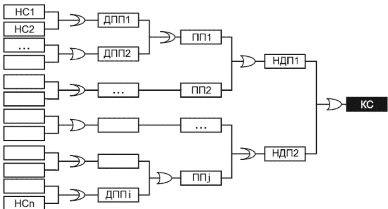
Рисунок 2 - Структура дерева отказов
