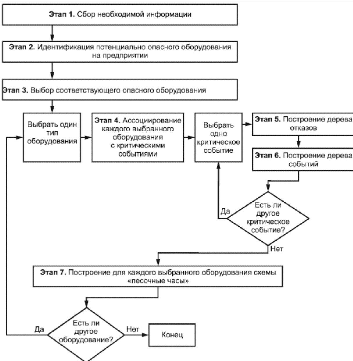
Рисунок 1 - Основные этапы МИСУИ
