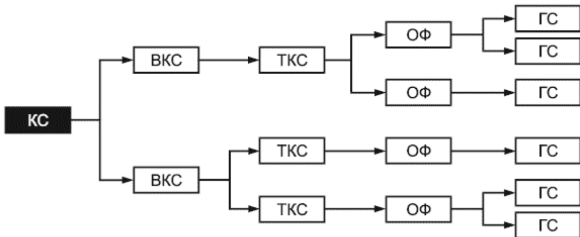
Рисунок 3 - Структура дерева событий
