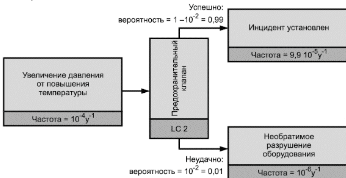
Рисунок 4 - Вероятность наступления событий в развернутом виде
