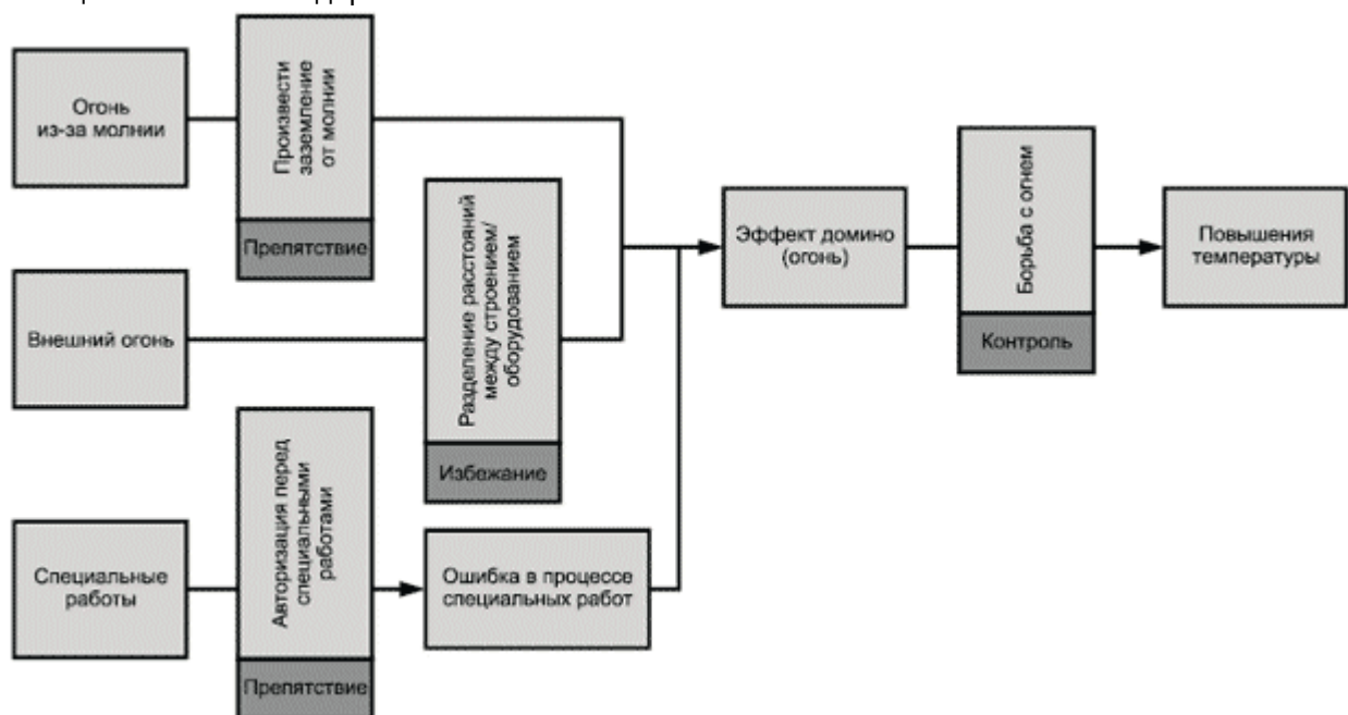
Рисунок 2 - Барьеры, размещенные на ветвях дерева отказов
