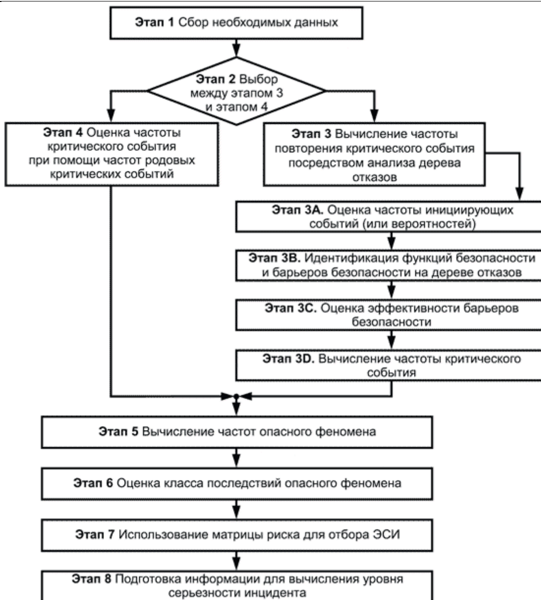
Рисунок 1 - Общая схема этапов МИЭСИ
