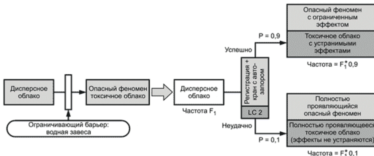
Рисунок 10 - Вероятность перехода событий с использованием барьера "Ограничение"
