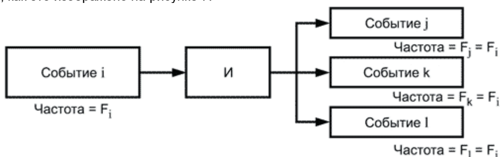
Рисунок 6 - Частота наступления каждого опасного события (ворота "И")
