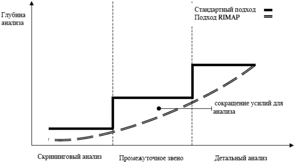
Рисунок 3 - Многоуровневый анализ риска. Уровень иерархии оборудования или компонента Входные данные для скрининга и детального анализа, обычно необходимые для каждого этапа оценки риска, приведены в таблице 3. Можно заметить, что некоторые входные данные характерны для обоих видов анализа, при этом для детального анализа требуются более сложные данные.
