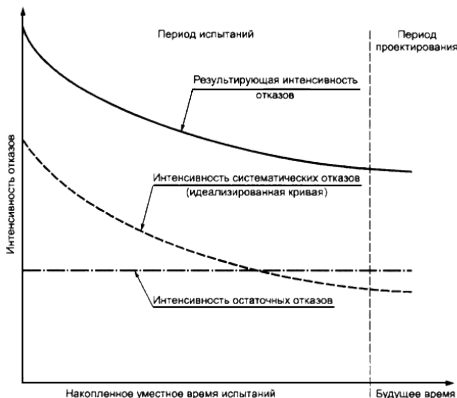
Рисунок 11 - Прогнозируемый параметр потока отказов, оцененный с помощью моделирования 6.4.8.4 Другие оценки
