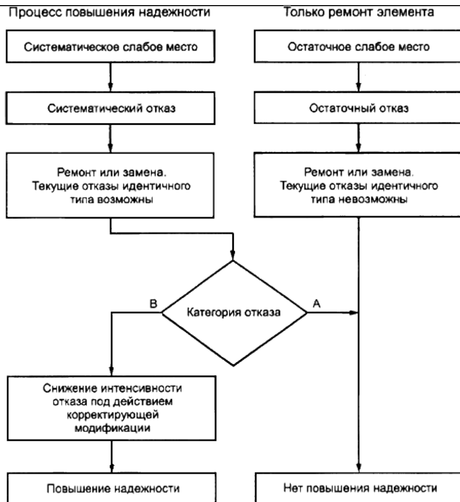
Рисунок 1 - Сравнение процесса повышения надежности и ремонта
