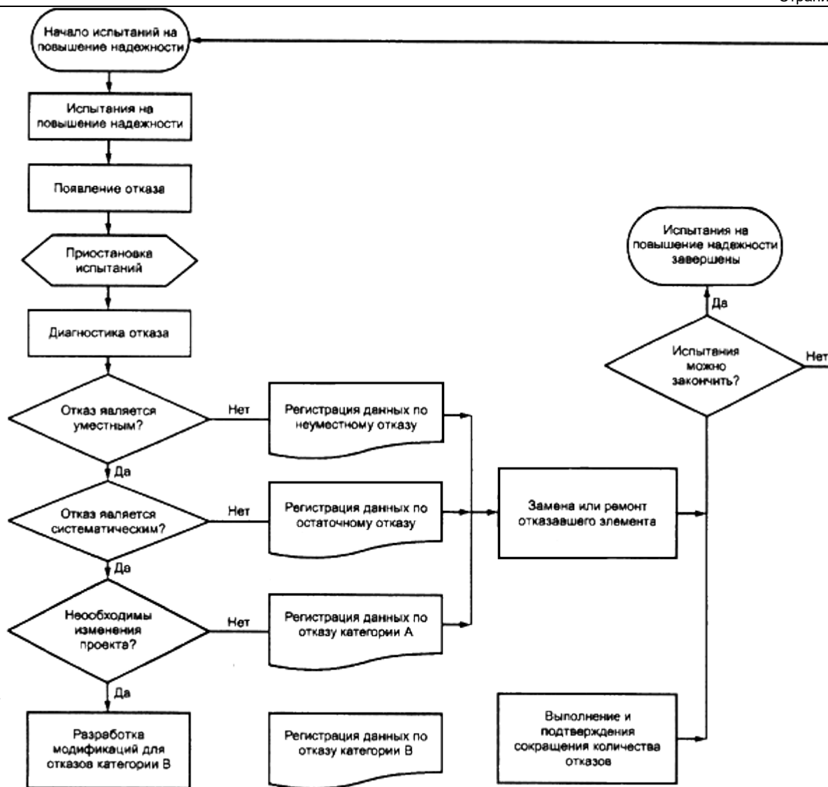
Рисунок 8 - Процесс испытаний на повышение надежности 6.4.4.3 Категории уместных отказов
