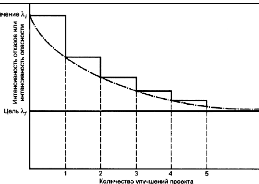
Рисунок 2 - Запланированное улучшение (снижение) эквивалентной интенсивности отказов По оси абсцисс отложены периоды времени до улучшения проекта. Полное время - это весь период проектирования.
