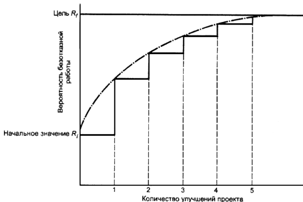
Рисунок 3 - Запланированное улучшение вероятности безотказной работы 4.5.3 Повышение надежности в ходе программы испытаний
