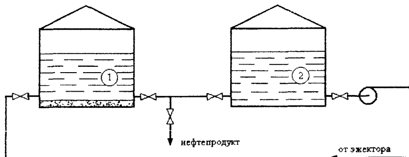
Рисунок 15 - Схема каскадного отстойника их двух РВС
