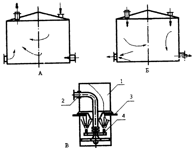
1 - цилиндрический корпус; 2 - паропроводящая труба; 3 - опорный лист пароежектора; 4 - ротор с двумя соплами
