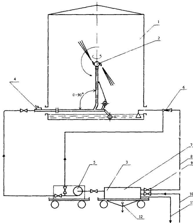
1 - зачищаемый резервуар; 2 - машинка моечная; 3 - тележка; 4 - лебедка; 5 - насос моещей воды; 6 - эжектор; 7 - отстойник; 8 - рукав соединительный; 9 - задвижка; 10 - пожарный водопровод; 11 - промливневая канализация; 12 - выпуск шлама
