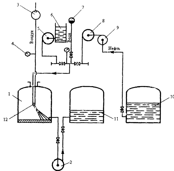
1 - очищаемый резервуар; 2 - откачивающий насос; 3 - компрессор; 4 - манометр; 5 - дозировочный насос; 6 - емкость для водного раствора объемом 5 м 3 ; 7 - пожарный гидрант, 8 - агрегат ПНА для закачки нефти; 9 - подпорный насос; 10 - резервуар с нефтью; 11 - резервуар-отстойник; 12 - моечная машинка ММС-100
