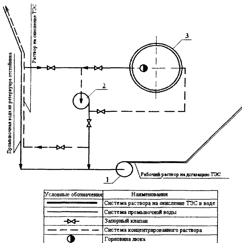
1 - насос промывочной воды; 2 - насос приготовления раствора; 3 - цистерна раствора
