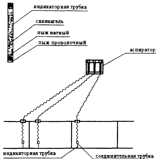
Рисунок 19 - Схема отбора пробы воздуха на содержание ТЭС
