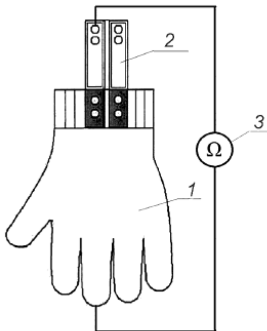
1 - защитная перчатка; 2 - контактный вывод; 3 - омметр
