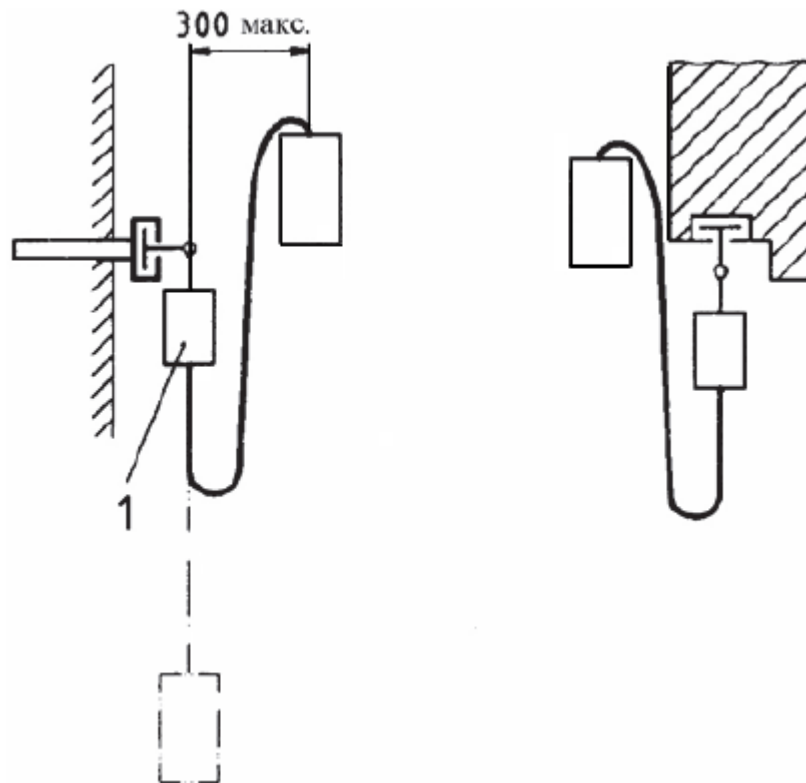
1 - устройство измерения силы
