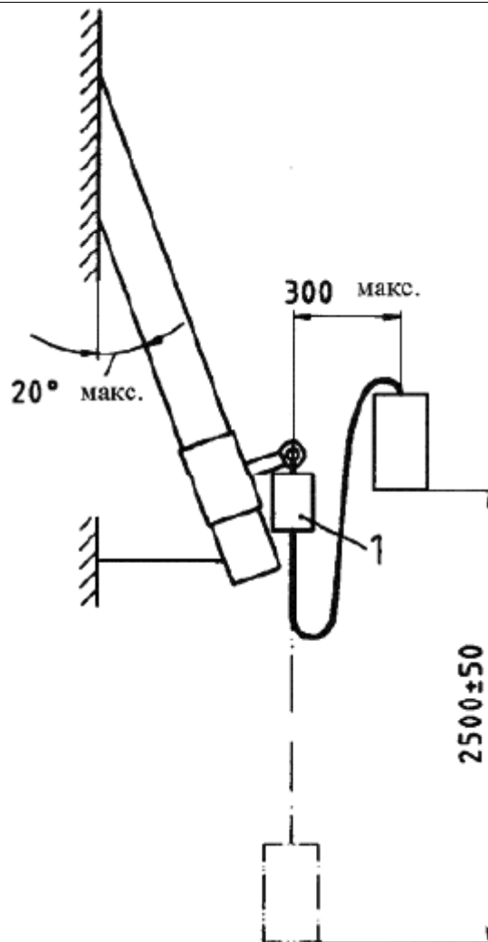
1 - устройство измерения силы
