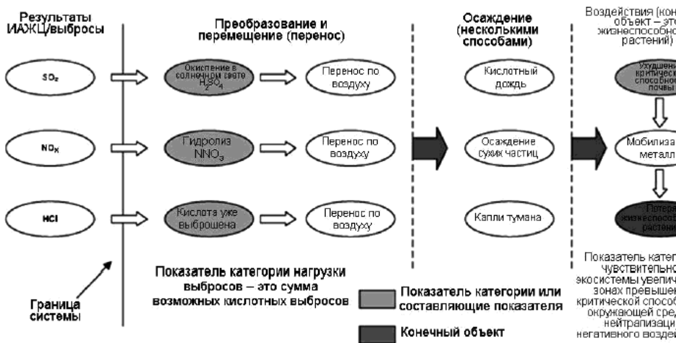
Рисунок 6 - Упрощенный экологический механизм закисления
