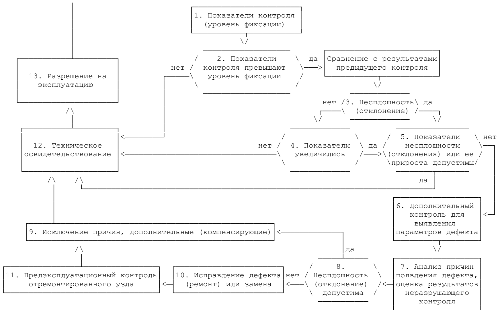
Рис. 14.1. Схема принятия решения и оценка допустимости несплошности при проведении эксплуатационного контроля металла оборудования, трубопроводов других элементов АС
