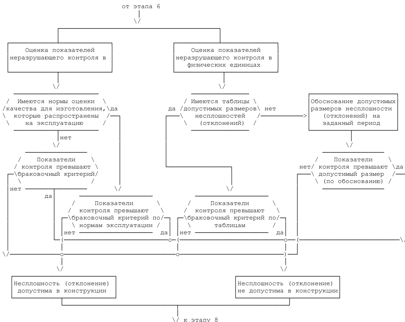
Рис. 14.2. Схема принятия решения и оценка допустимости несплошности при проведении эксплуатационного контроля металла оборудования, трубопроводов других элементов АС (расшифровка этапа 7 на рис. 14.1 настоящего приложения)
