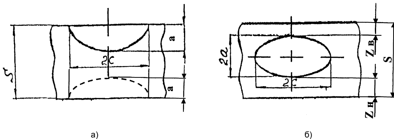
Рис. 9.1. Несплошности, ориентированные в продольном направлении (вдоль продольной оси оборудования или трубопровода, или поперек сварного соединения): а) поверхностная несплошность, б) подповерхностная несплошность
