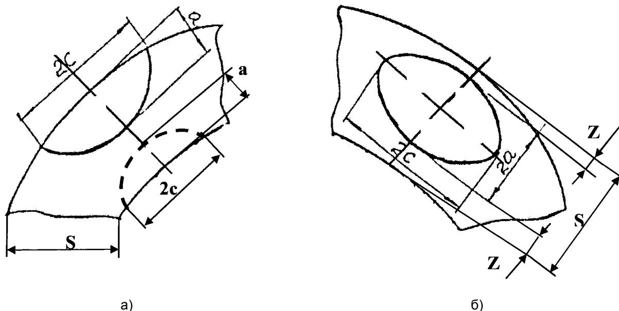
Рис. 9.2. Несплошности, ориентированные в кольцевом направлении (поперек продольной оси оборудования или трубопровода, или вдоль сварного соединения): а) поверхностная несплошность, б) подповерхностная несплошность
