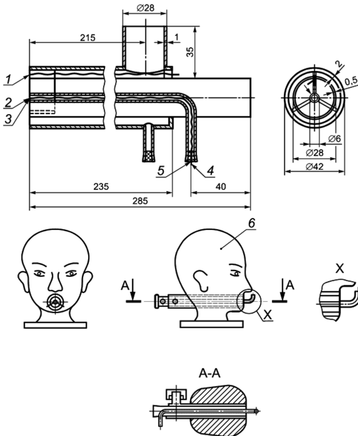
Рисунок А.2 - Тройник для самоспасателя с центральным резьбовым соединением
