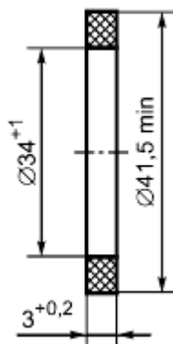
Рисунок Б.5 - Прокладка ДРУ
