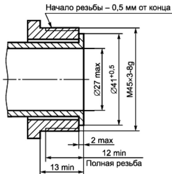
Рисунок Б.1 - Резьбовые соединения с внешней резьбой для систем с одним каналом подачи воздуха РПА
