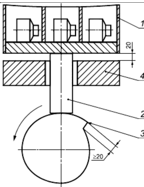
1 - стальная коробка; 2 - поршень; 3 - кулачок; 4 - стальная пластина
