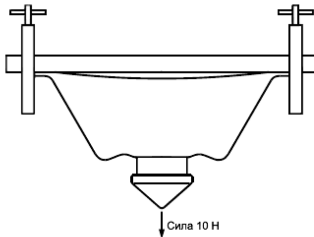
Рисунок 11 - Зажимное устройство для лицевой части
