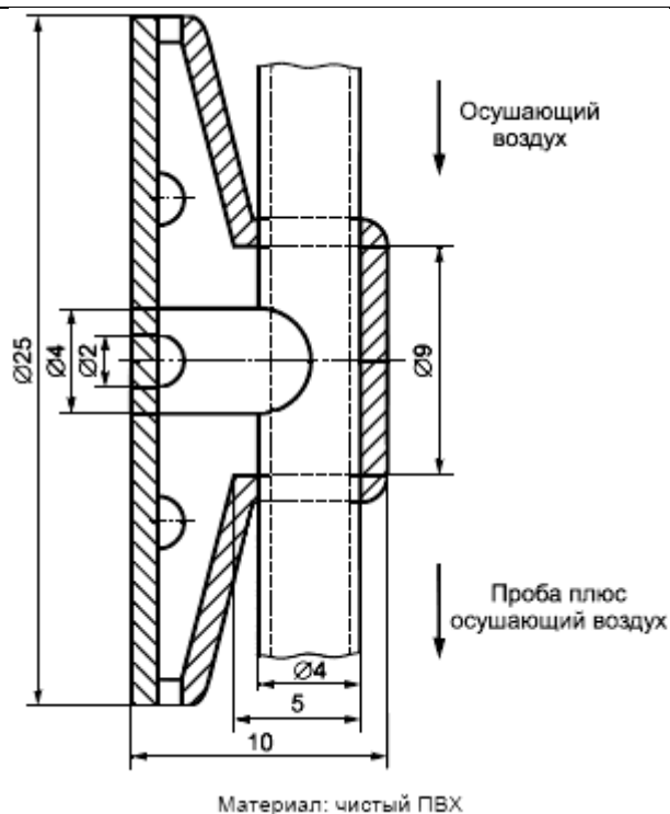
Рисунок 5 - Пробоотборник
