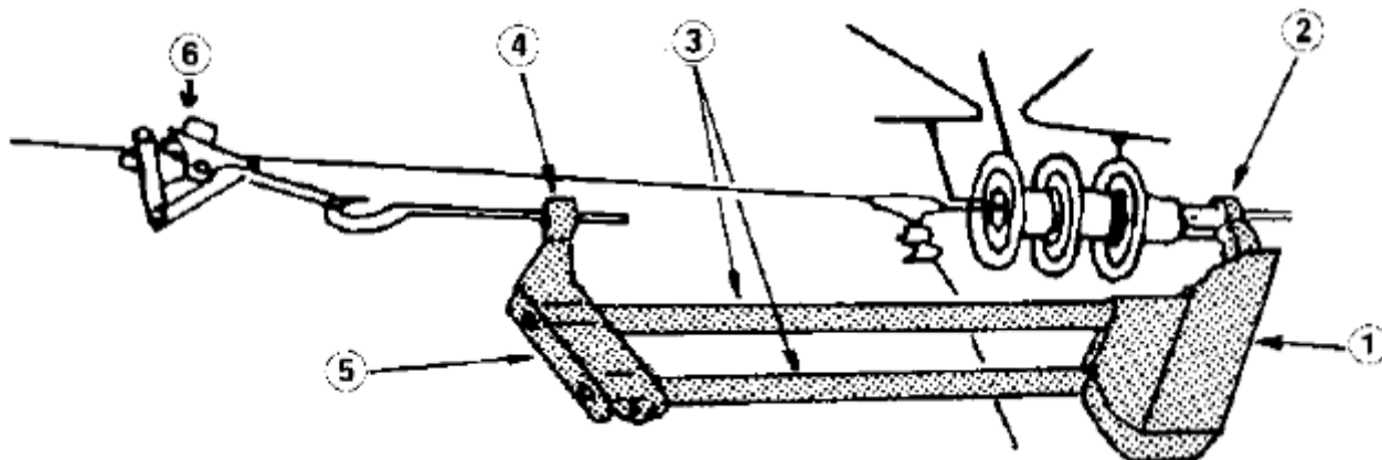
1 - боковина (с изолирующим покрытием); 2 - крюк; 3 - диэлектрические трубки; 4 - винтовой домкрат; 5 - боковина; 6 - натяжные монтажные зажимы (зажимы для троса) [IEC 60050-651:651-22-26]
