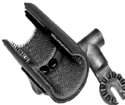
Полутрубчатая щетка
