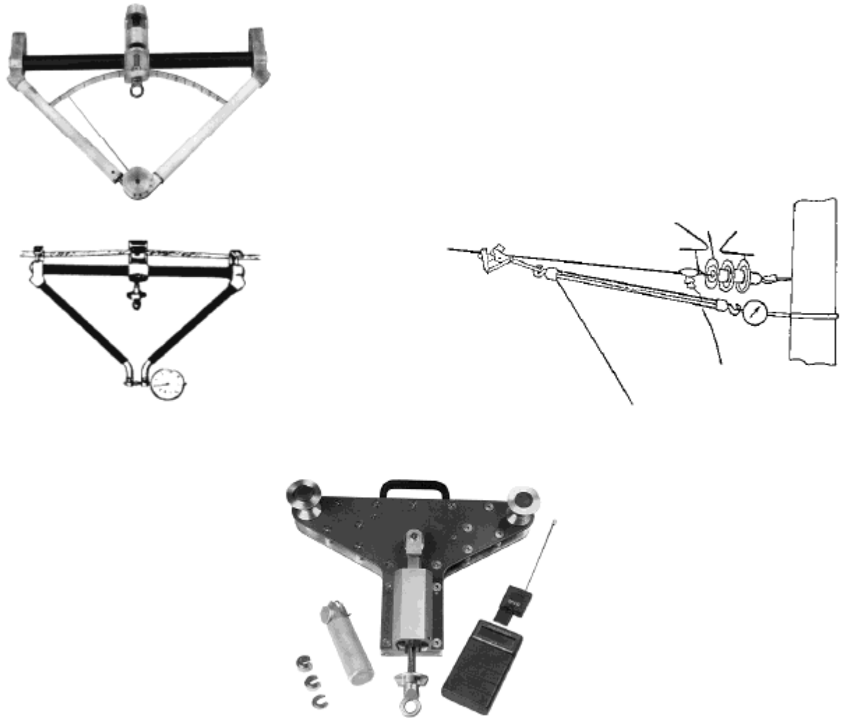
Различные конструкции динамометров
