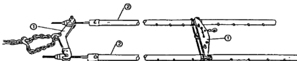
1 - нагрузочное коромысло; 2 - регулируемая тяга
