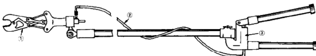
1 - режущая головка; 2 - гибкий шланг; 3 - гидронасос
