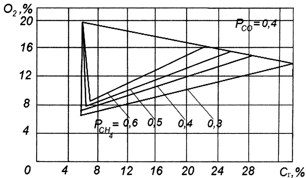
Рис. 5. Треугольник взрываемости при P_{CO} = 0,4
