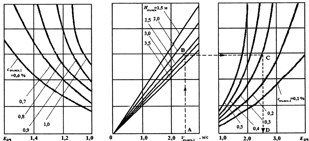
Рис. 7. Номограмма для определения K_{оч}
