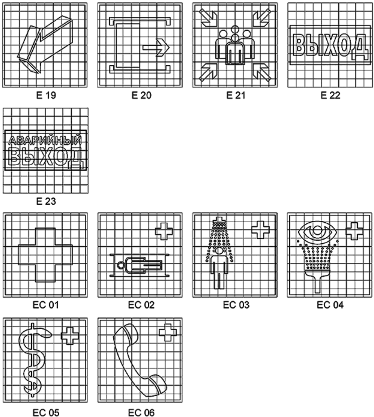
Рисунок П.5, лист 1 - Эвакуационные знаки и знаки медицинского и санитарного назначения
