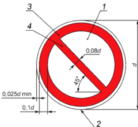
d - диаметр круга; 1 - основная поверхность; 2 - кант; 3 - кайма; 4 - поперечная полоса Рисунок 1* - Основа цветографического изображения и соотношение размеров запрещающих знаков безопасности
