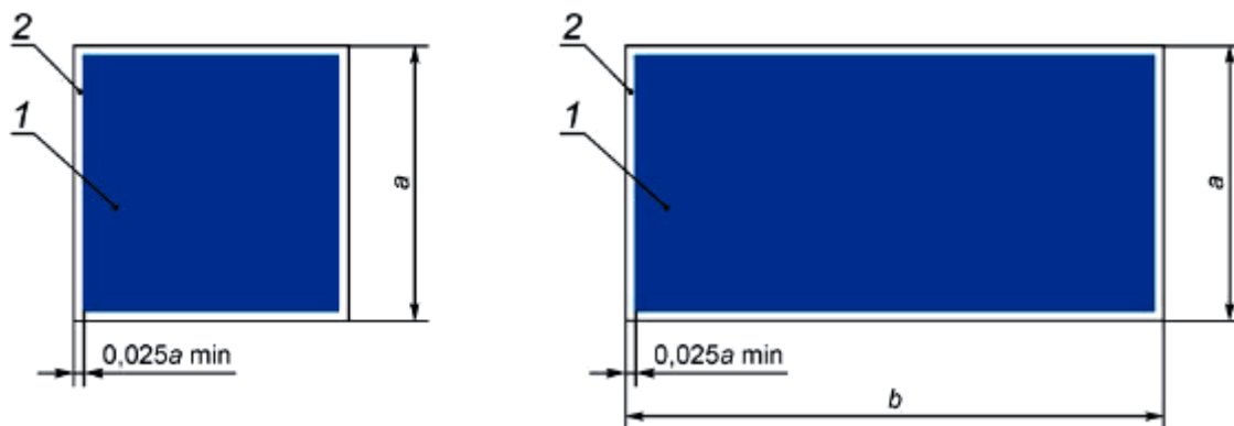
a, b - стороны квадрата и прямоугольника ( 2a = b ); 1 - основная поверхность; 2 - кант Рисунок 6 - Основа цветографического изображения и соотношение размеров указательных знаков безопасности
