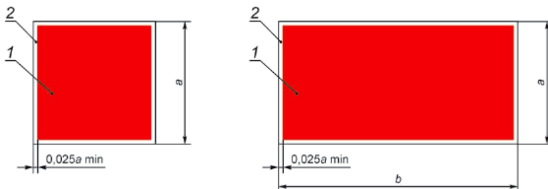
a, b - стороны квадрата и прямоугольника ( 2a = b ); 1 - основная поверхность; 2 - кант Рисунок 4 - Основа цветографического изображения и соотношение размеров знаков пожарной безопасности
