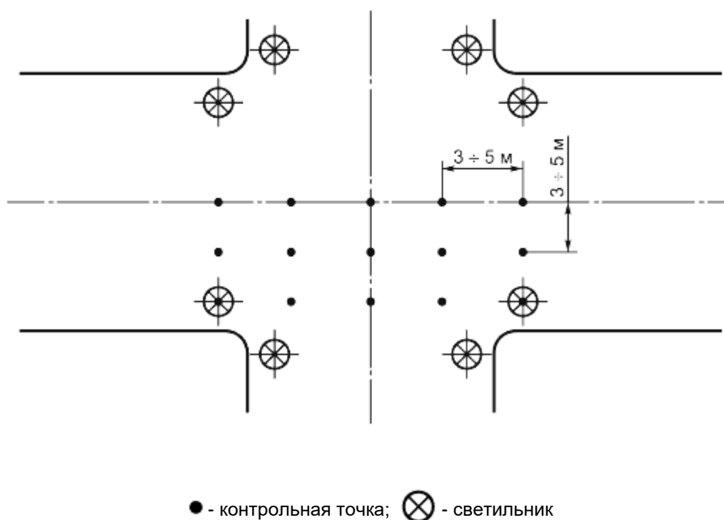
Рисунок Б.5 - Расположение контрольных точек при измерении средней освещенности улиц на перекрестке
