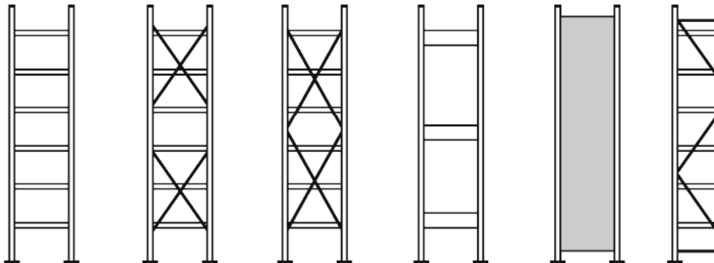
Рисунок 1 - Варианты рам стеллажей с элементами жесткости
