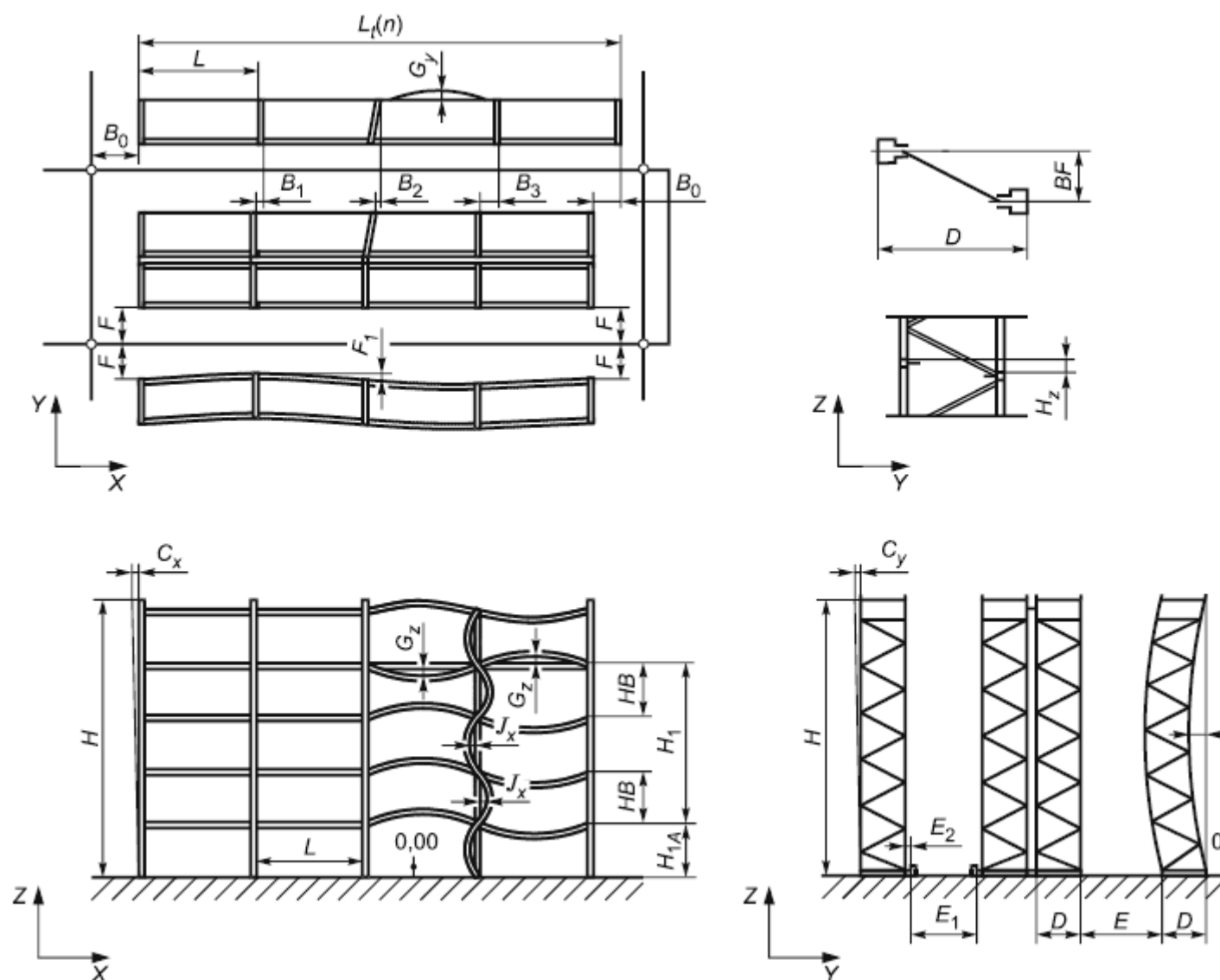
Рисунок 7 - Параметры, подлежащие контролю в ненагруженном состоянии системы Таблица 1 - Допуски, отклонения и деформации
