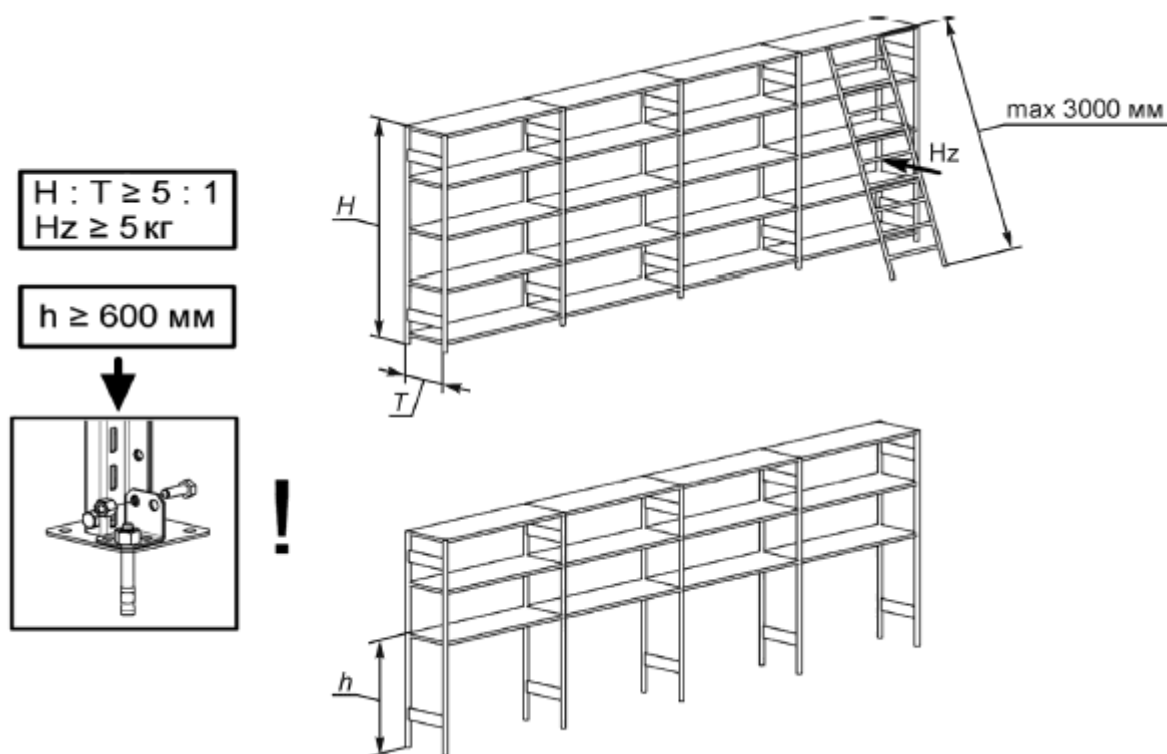
Рисунок 11 - Требования по креплению стеллажа к полу
