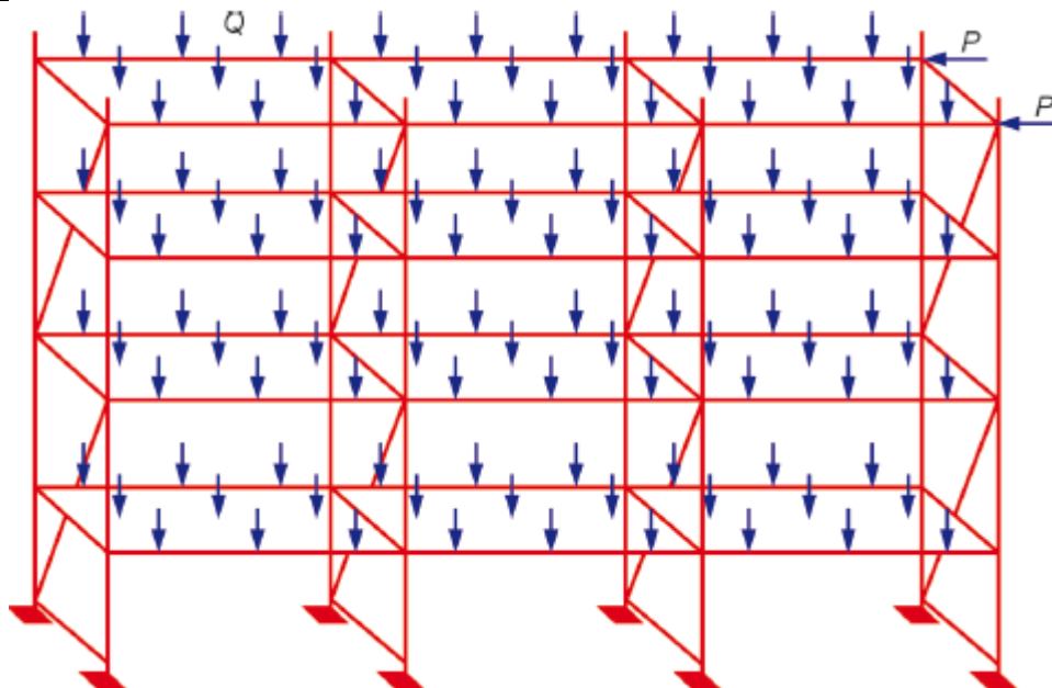
Рисунок 9 - Испытание на воздействие горизонтальной нагрузки
