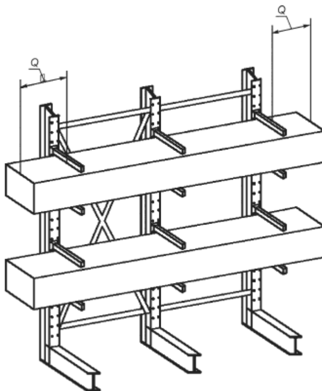
Рисунок 12 - Размещение грузов на консольных стеллажах На консоли стеллажей допускается только равномерно распределенная статическая нагрузка
