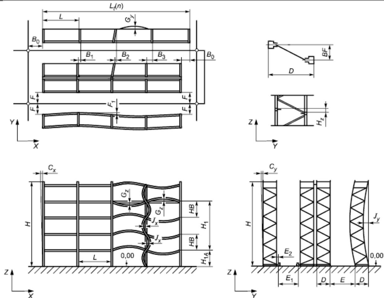
Рисунок 8 - Параметры, подлежащие контролю в ненагруженном состоянии системы Таблица 4 - Допуски, отклонения и деформации в ненагруженном состоянии стеллажа
