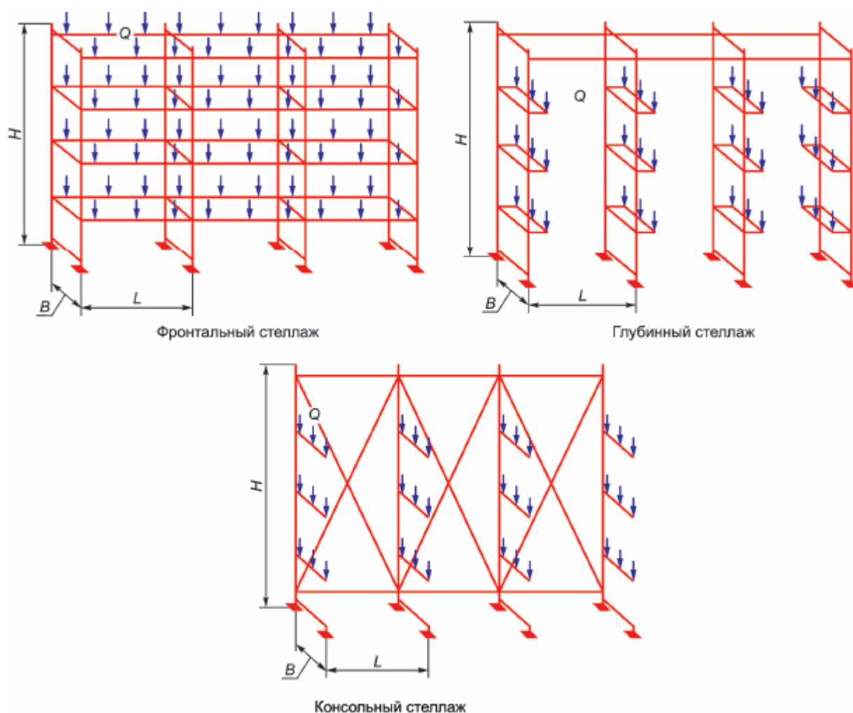
Рисунок 15 - Методы испытаний на воздействие вертикальной нагрузки
