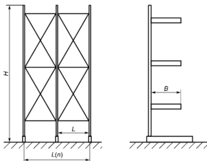
Рисунок 2 - Общий вид набивного (глубинного) стеллажа
