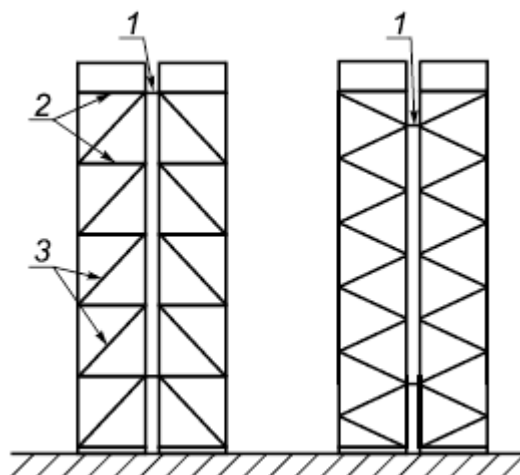
1 - межрамная связь; 2, 3 - элементы раскосной системы
