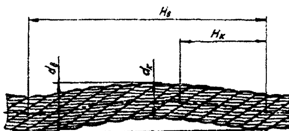
Рисунок 9. Волнистость каната
