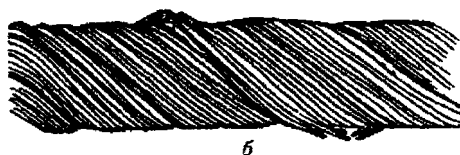
Рисунок 2. Сочетание обрывов проволок с их износом: а - в канате крестовой свивки; б - в канате односторонней свивки
