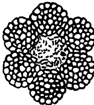
Рисунок 7. Местное уменьшение диаметра каната на месте разрушения органического сердечника
