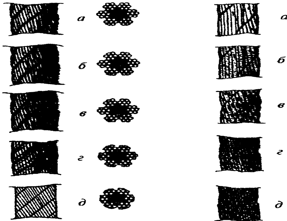
Рисунок 5. Износ наружных проволок каната крестовой свивки:
