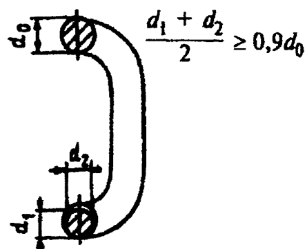
Рисунок 2 Уменьшение диаметра сечения звена цепи: d_0 - первоначальный диаметр, мм; d_1, d_2 - фактические диаметры сечения звена, измеренные во взаимно перпендикулярных направлениях, мм
