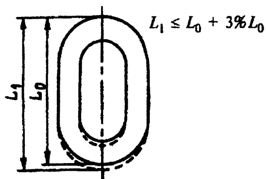
Рисунок 1 Увеличение звена цепи: L_0 - первоначальная длина звена, мм; L_1 - увеличенная длина звена, мм
