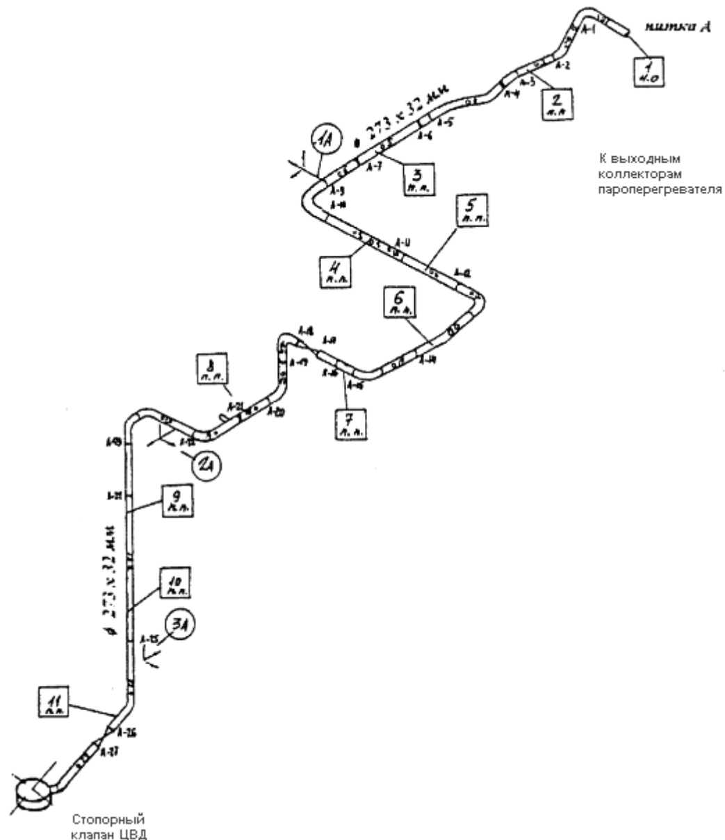
Схема паропровода
