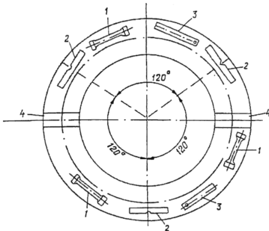
Рис.1. Схема вырезки образцов из трубы паропровода: 1 и 2 - образцы для испытания на разрыв и удар соответственно; 3 - образец для карбидного анализа;
