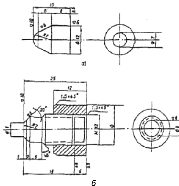
Рис.3. Эскиз репера:
