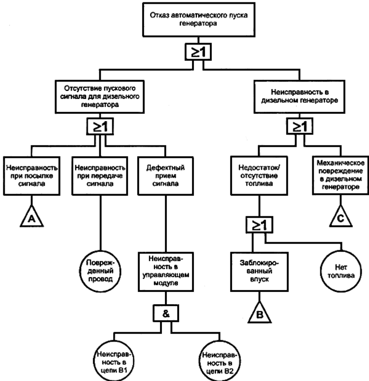
Рисунок А.1 - Пример "дерева неисправностей"
