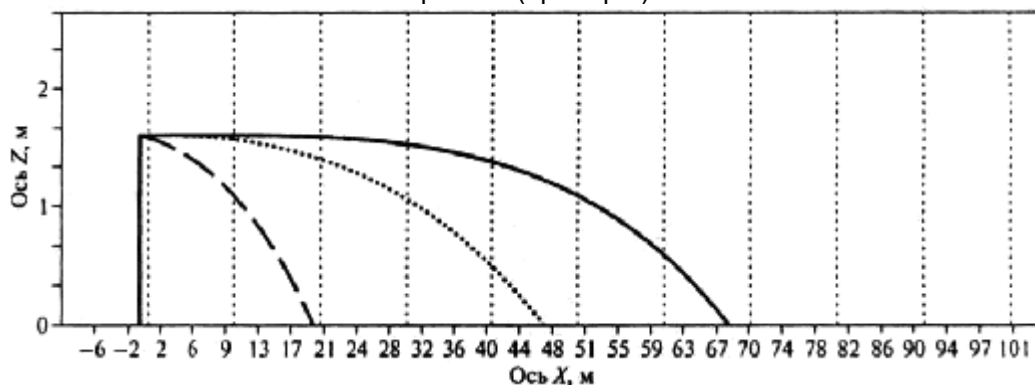
Рис.9.9. Зоны достижения концентраций ВКПВ, НКПВ и 0,5НКПВ на поверхности земли при выбросе пропана (пример 4)
