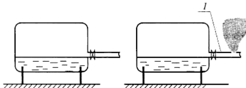
Рис.4.8. Разгерметизация трубопровода с газовой фазой, присоединенного к емкости (1 - отсекаемый участок аварийного трубопровода) (сценарий 4)
