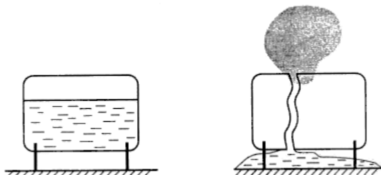
Рис.4.2. Мгновенное разрушение емкости с жидкой фазой (сценарий 3)
