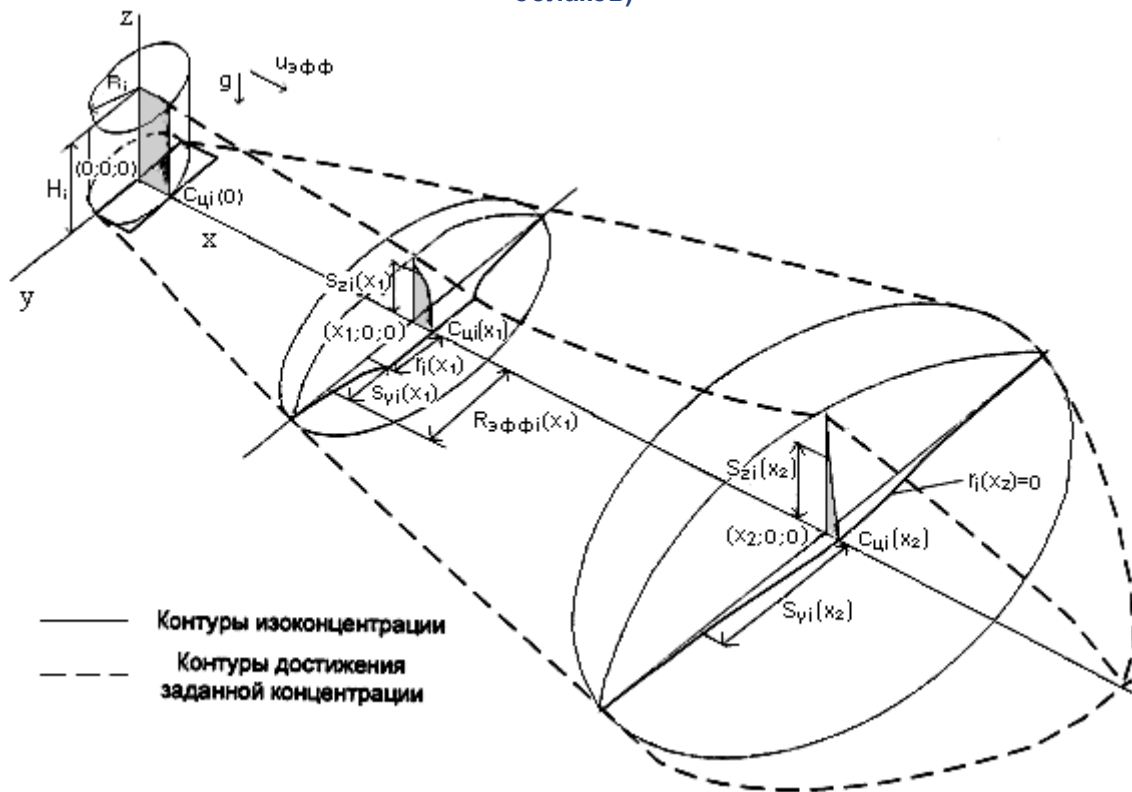
Рис.3.1. Схема распространения первичного облака
