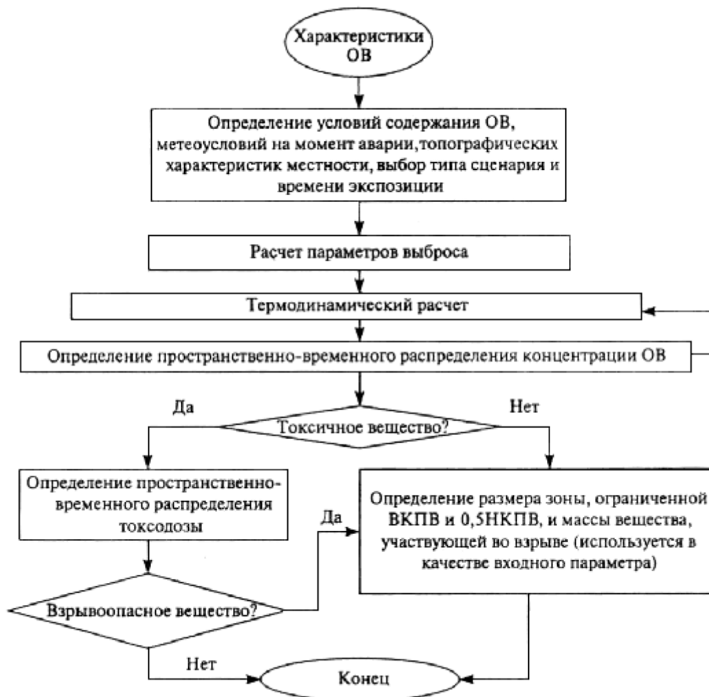
Рис.10.1. Блок-схема расчета последствий аварийного выброса опасных веществ
