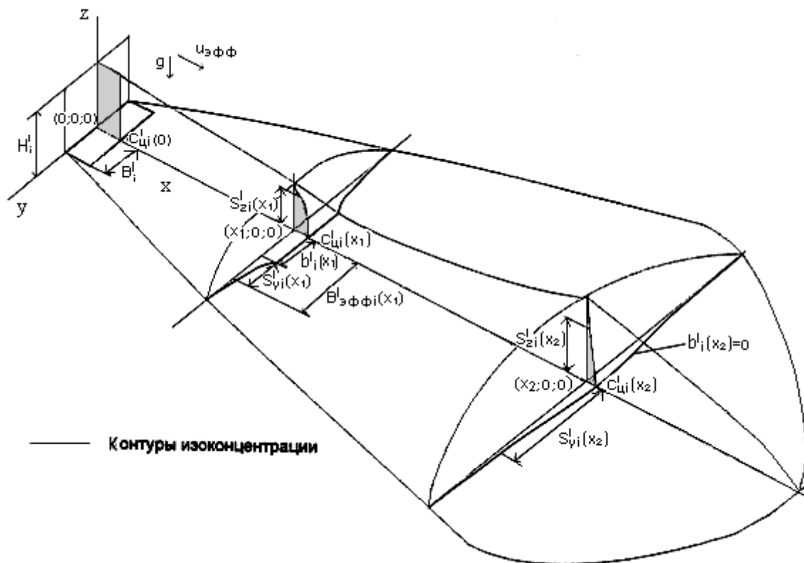
Рис.3.2. Схема распространения вторичного облака
