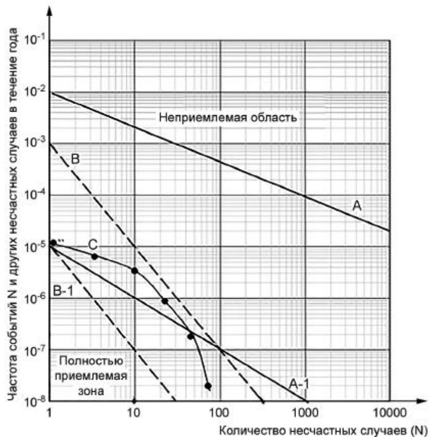
Рисунок Б.15 - Пример диаграммы F-N
