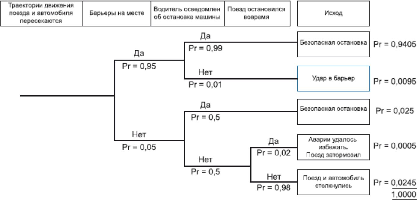
Рисунок Б.4 - Пример анализа дерева событий
