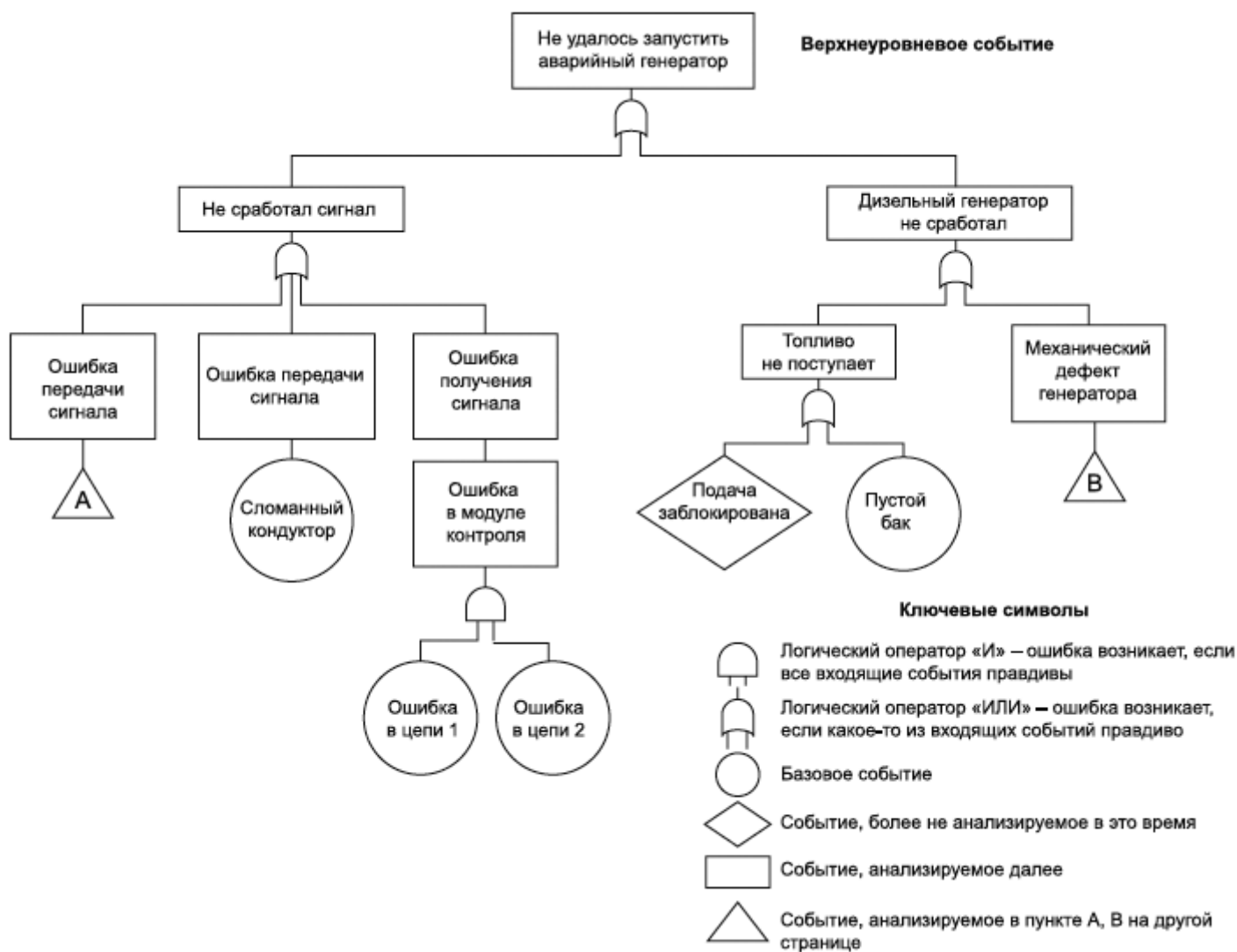
Рисунок Б.5 - Пример дерева отказов
