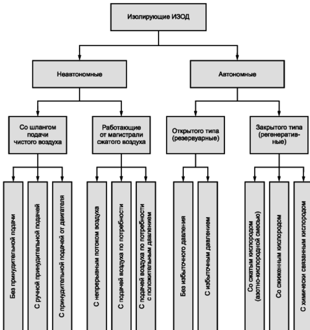
Рисунок 4 - Классификация изолирующих СИЗОД по конструкции и принципу действия 3.1.3.2 Изолирующие СИЗОД по назначению подразделяют на:
