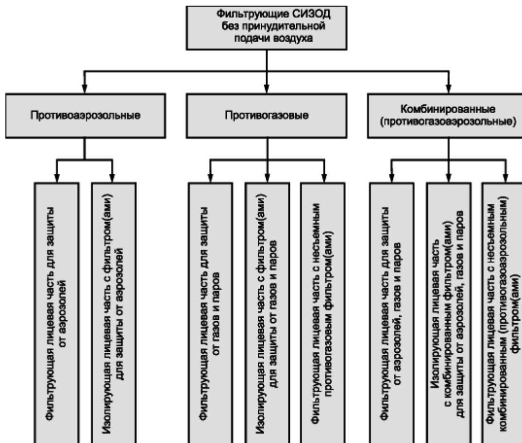
Рисунок 2 - Классификация фильтрующих СИЗОД без принудительной подачи воздуха по конструкции и назначению
