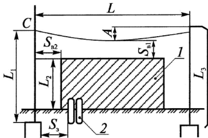
Рисунок 2. Отдельно стоящий тросовый молниеотвод: L - расстояние между молниеотводами; L_1 , L_3 - протяженность токопроводов; L_2 - высота защищаемого сооружения; S_{\text{г1}} , S_{\text{г2}} - наименьшие допустимые расстояния от тросового молниеотвода соответственно в точках А и С до защищаемого сооружения; S_{\text{з}} - наименьшее допустимое расстояние от заземления до металлических коммуникаций; 1 - защищаемое сооружение; 2 - металлические коммуникации
