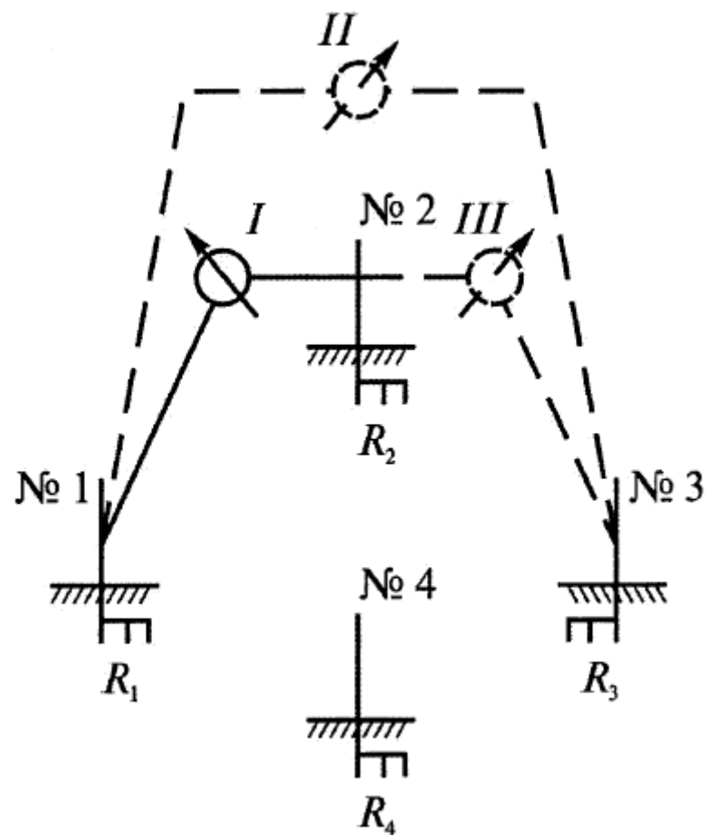
Рисунок 17. Схема измерения сопротивления заземлителей способом трех измерений
