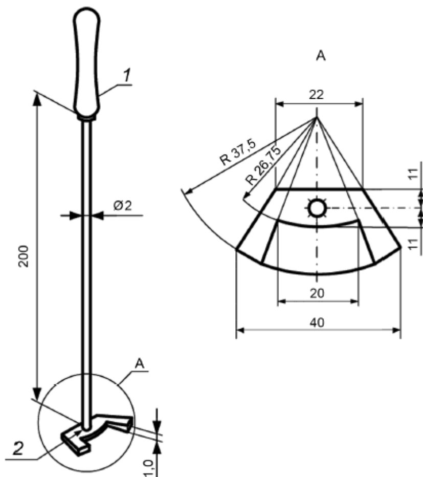
Рисунок 6.4 - Шаблон для установки и контроля печного термоэлектрического преобразователя
