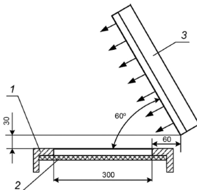
1 - держатель с образцом; 2 - образец; 3 - электрическая радиационная панель Рисунок 12.2 - Взаимное расположение радиационной панели и держателя с образцом
