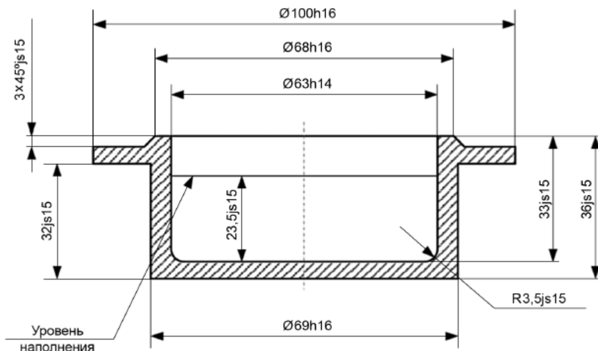
Рисунок 30.1 - Открытый тигель Кливленда
