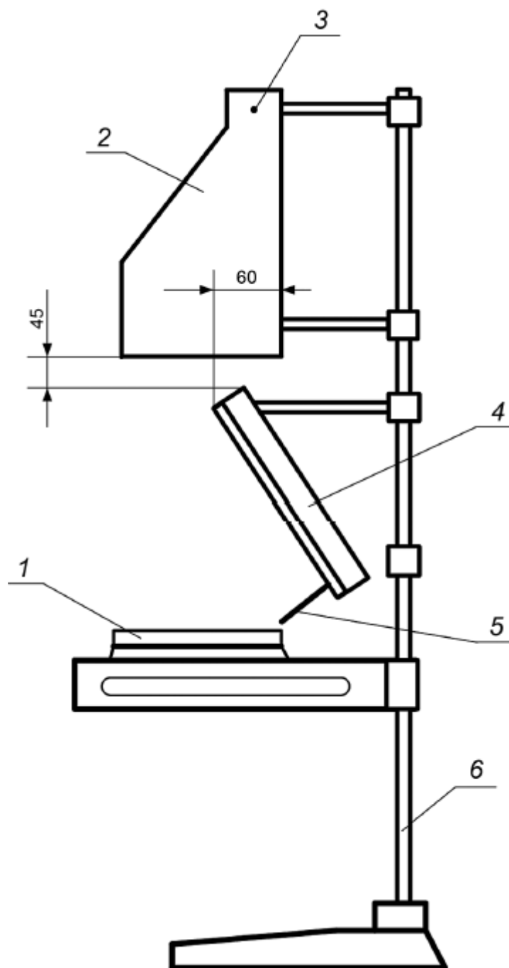
1 - держатель образца; 2 - вытяжной зонт; 3 - термоэлектрический преобразователь; 4 - электрическая радиационная панель; 5 - газовая горелка; 6 - вертикальная стойка на опоре Рисунок 12.1 - Общий вид установки для определения линейной скорости распространения пламени Примечание - В качестве устройства, регулирующего расход газа, может использоваться расходомер типа ротаметр или аналогичный прибор с диапазоном, обеспечивающим требования 12.4.3.
