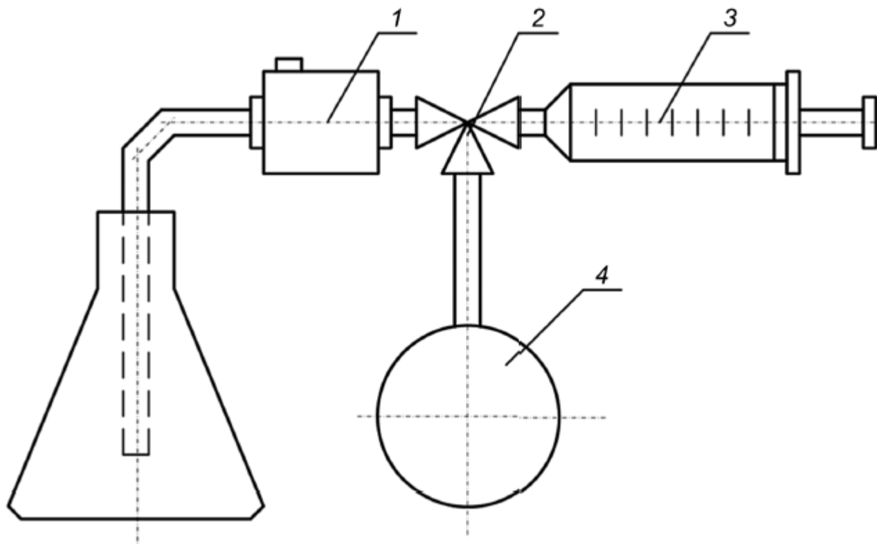
Рисунок 31.2 - Схема дозированной подачи газов
