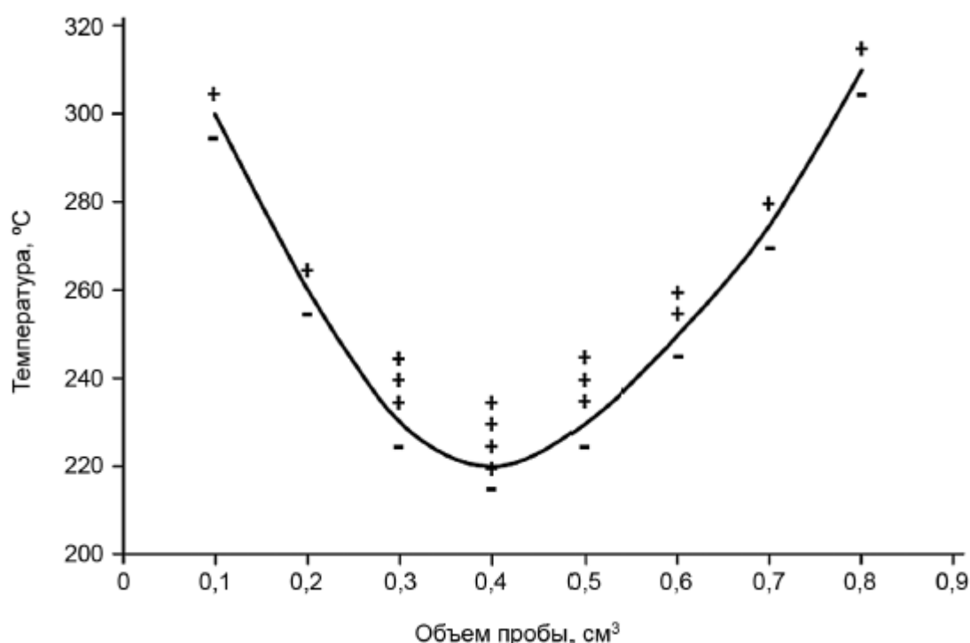
Рисунок 31.3 - График зависимости температуры самовоспламенения от объема пробы
