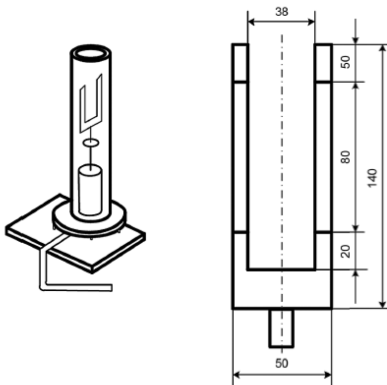
Рисунок 10.2 - Реакционная камера и рамка - держатель образца
