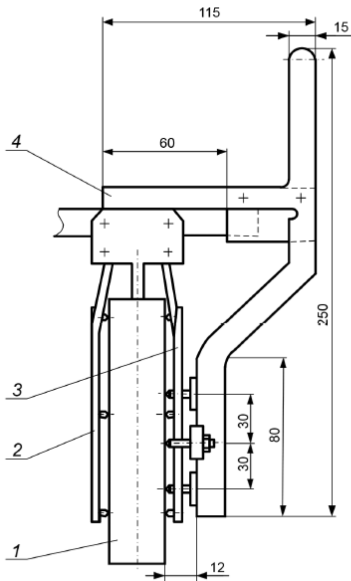
1 - образец; 2, 3 - держатели образца; 4 - шаблон Рисунок 7.2 - Шаблон
