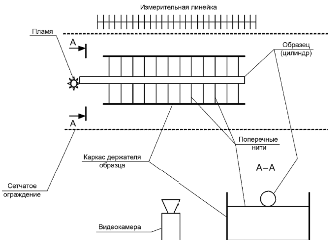
Рисунок 23.1 - Общий вид установки для определения нормальной скорости распространения пламени по аэровзвеси
