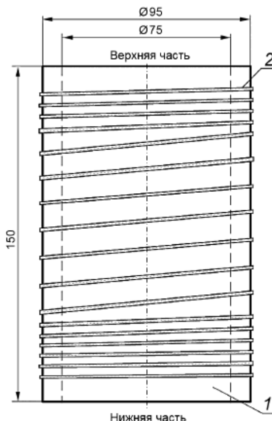
1 - трубчатая печь; 2 - нагревательный элемент
