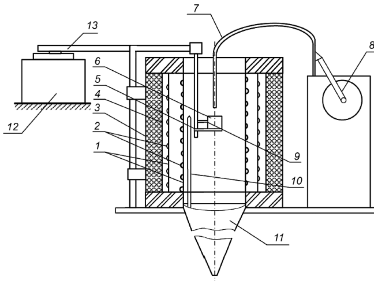
Рисунок 17.1 - Общий вид установки для определения удельной массовой скорости выгорания твердых веществ и материалов
