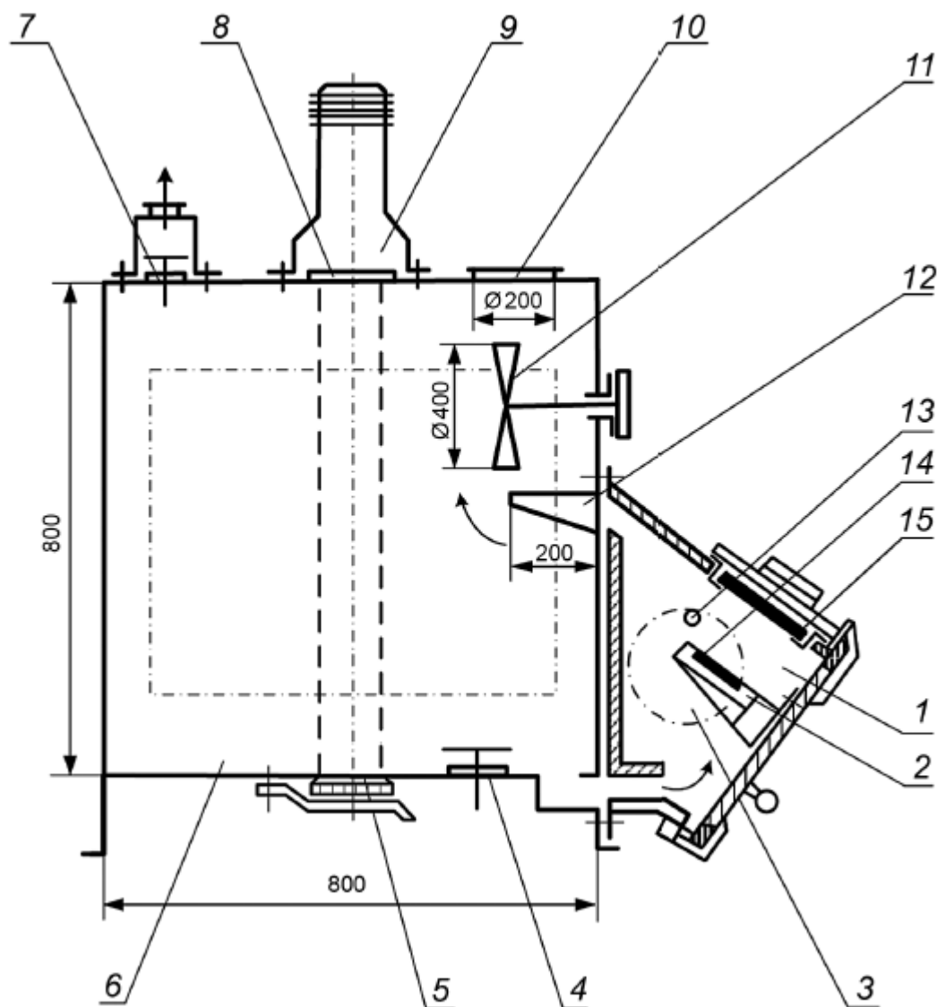
1 - камера сгорания; 2 - держатель образца; 3 - окно из кварцевого стекла; 4, 7 - клапаны продувки; 5 - приемник света; 6 - камера измерений; 8 - кварцевое стекло; 9 - источник света; 10 -
