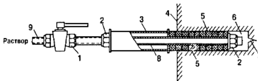
Рис.1. Установка иньектора в скважине:
