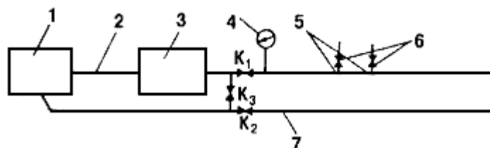
Рис.2. Принципиальная схема нагнетания цементного раствора:
