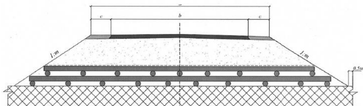
Рисунок П.10 - Конструкция земляного полотна на болотах III типа с двухрядным лежневым настилом и геополотном тканым
