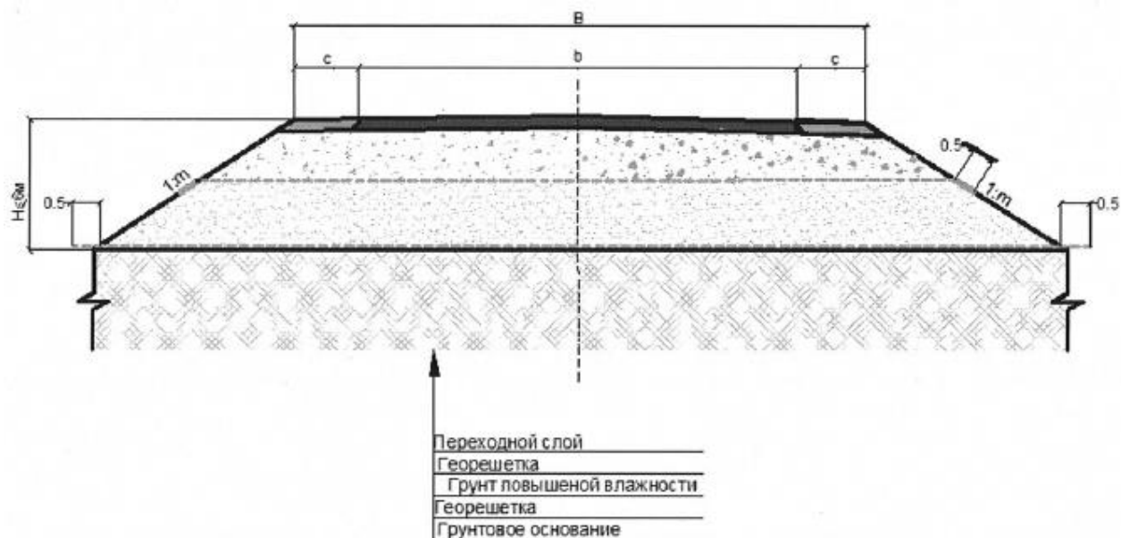
Рисунок П.8 - Земляное полотно высотой до 6 м из грунтов повышенной влажности с применением георешетки
