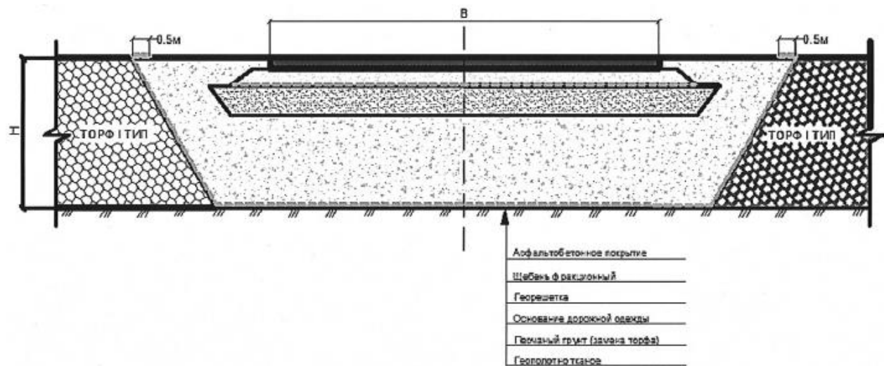
Рисунок П.6 - Земляное полотно с заменой пучинистого грунта с использованием геосинтетических материалов
