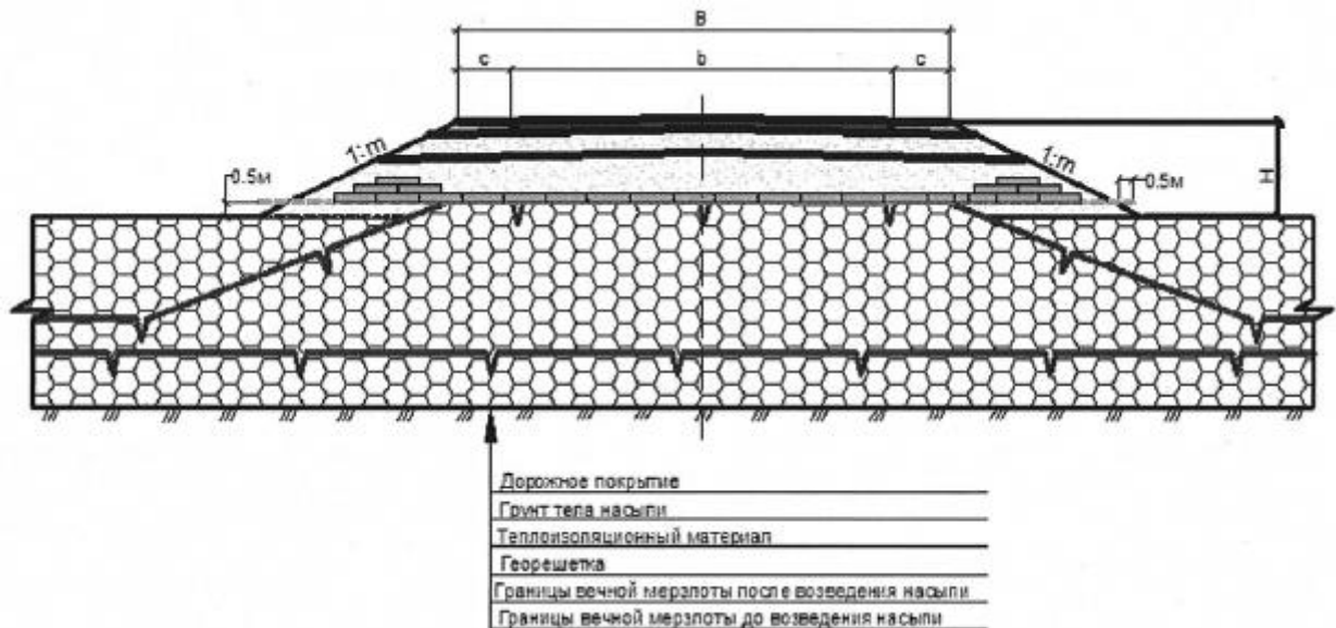
Рисунок П.4 - Земляное полотно с устройством теплоизолирующего слоя в зоне вечной мерзлоты и применением георешетки
