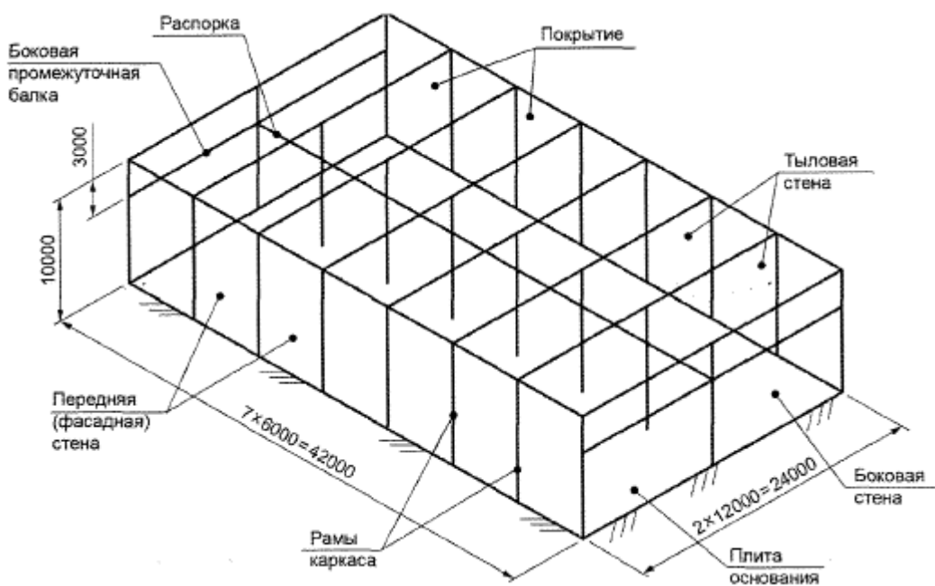
Рисунок М.3 - Расчетная схема здания, расположенного на расстоянии 80 м от эпицентра взрыва
