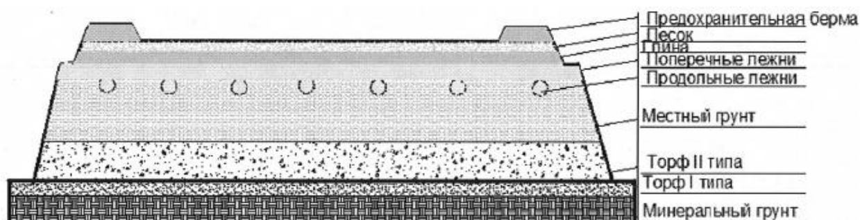
Рисунок П.11 - Конструкция земляного полотна на кустовой площадке скважин на болотах II типа
