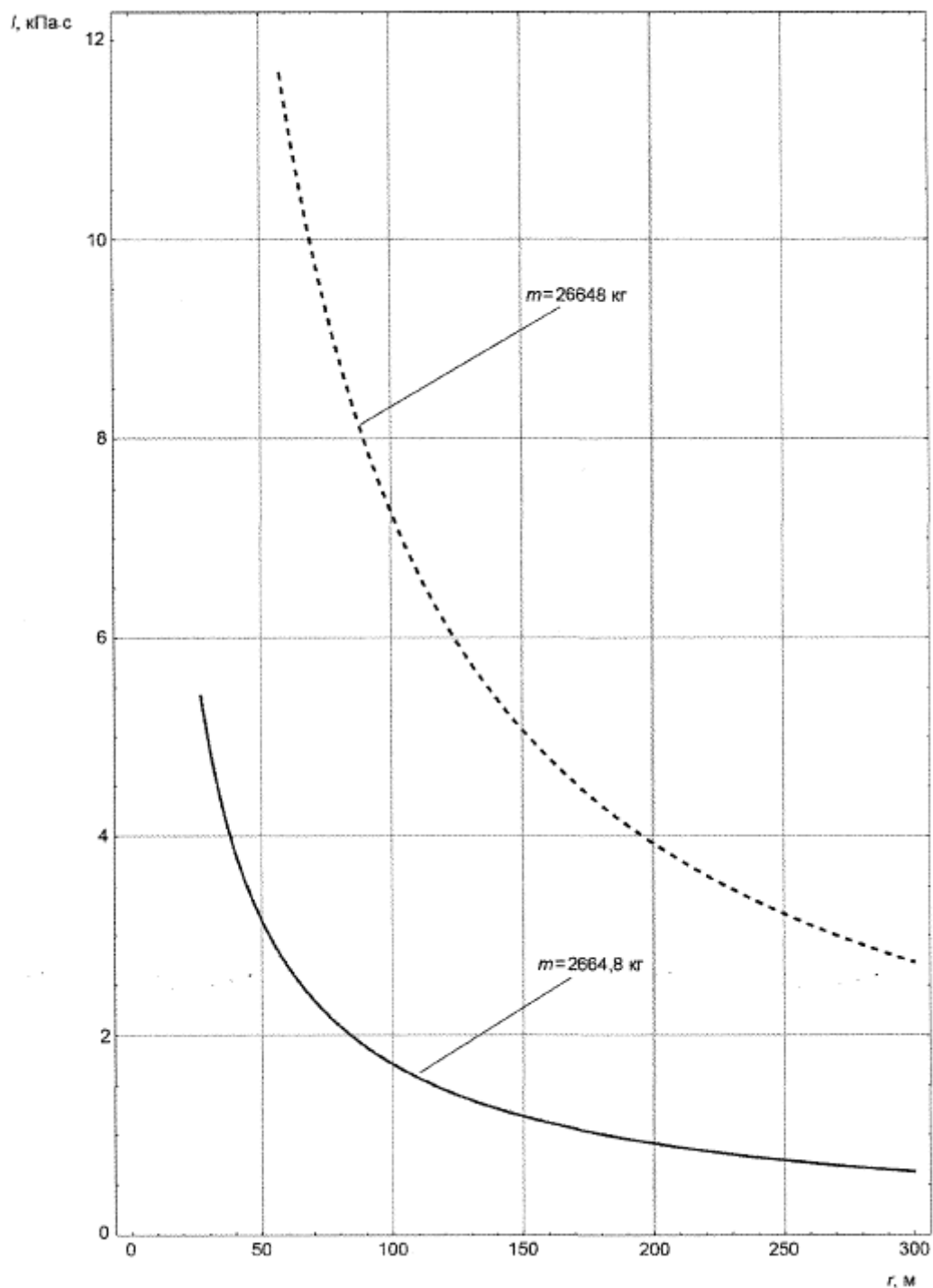
Рисунок Л.5 - Зависимость от расстояния до центра облака удельного импульса фазы сжатия воздушной ударной волны для различной массы пропана в облаке
