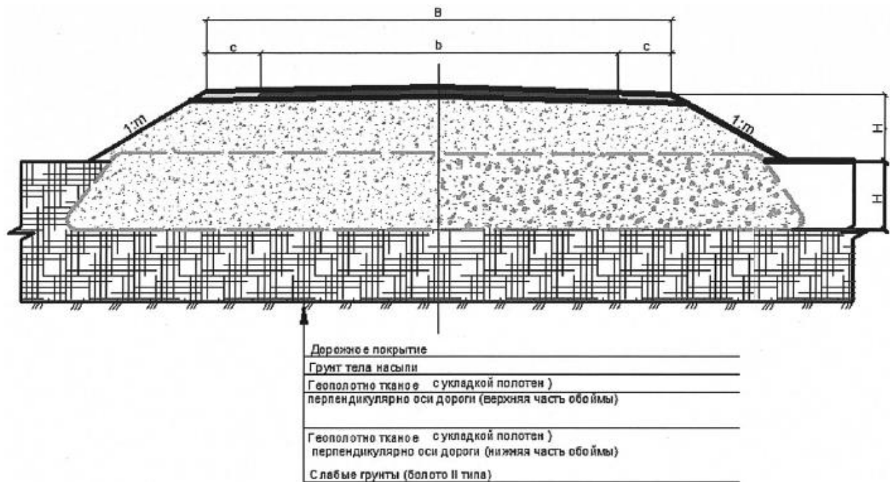
Рисунок П.5 - Насыпь на болотах II типа внутри обоймы из геосинтетических материалов
