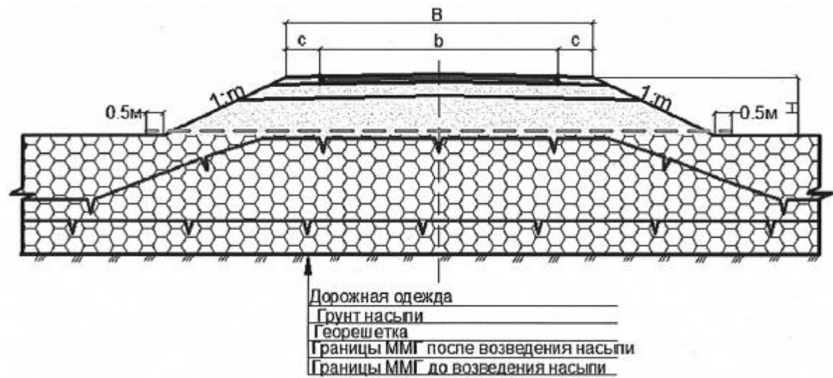
Рисунок П.3 - Земляное полотно на многолетнемерзлых грунтах с использованием георешетки
