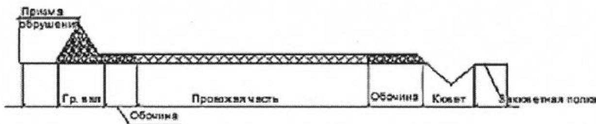
Рисунок 7.1а* - Поперечный разрез транспортной бермы
