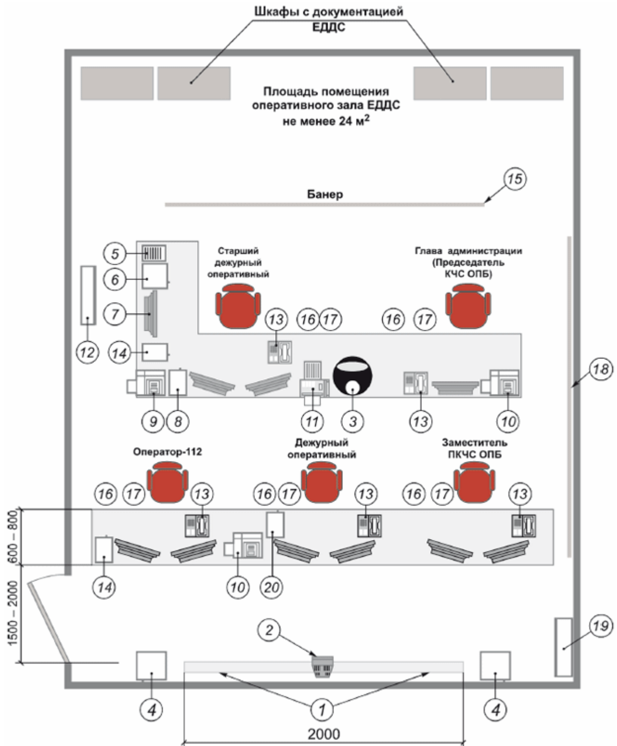
Рисунок А.1 - Примерная схема размещения рабочих мест и оборудования ЕДДС Условные обозначения оборудования и технических средств связи находящихся в оперативном зале ЕДДС (рисунок А.1):
