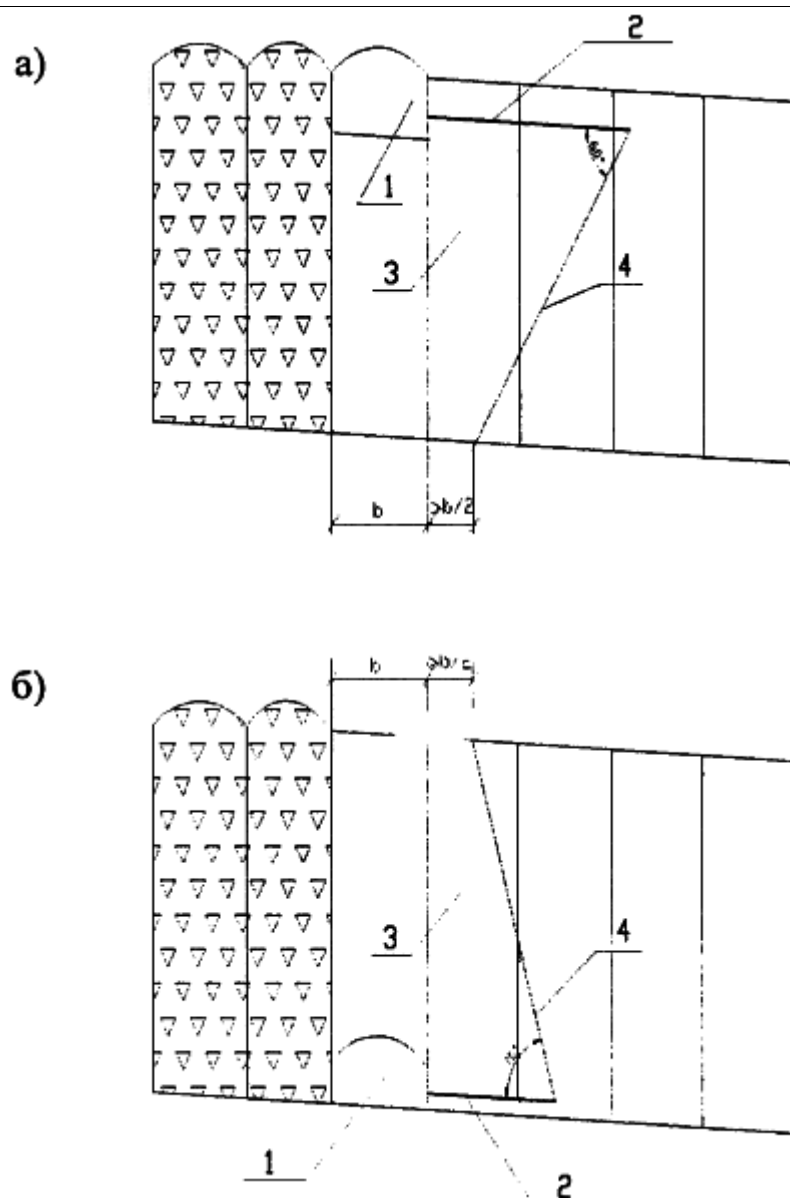
Рисунок 5 - Построение защищенной зоны бурением скважин большого диаметра по кровле (а) и почве (б) рудного тела
