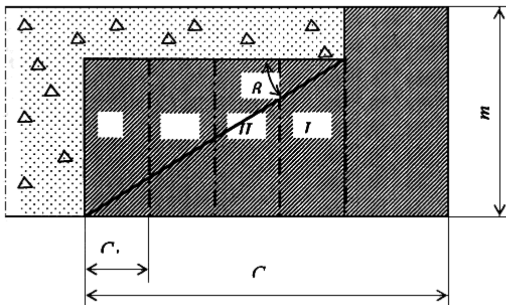
Рисунок 2 - Построение защищенной зоны при опережающей надработке рудного тела
