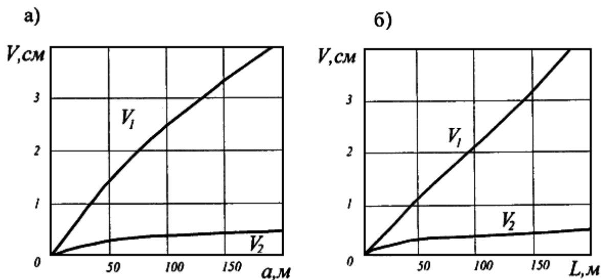
Рисунок 3 - Графики состояния целика
