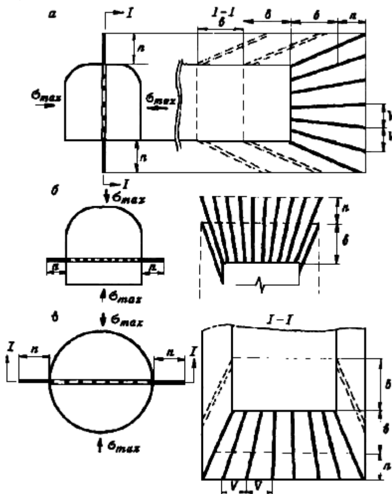
Рисунок 11 - Схемы камуфлетного взрывания по рядам шпуров:
