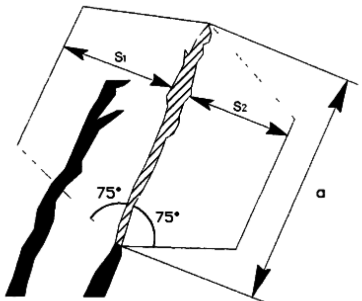
Рисунок 1 - Построение защищенной зоны
