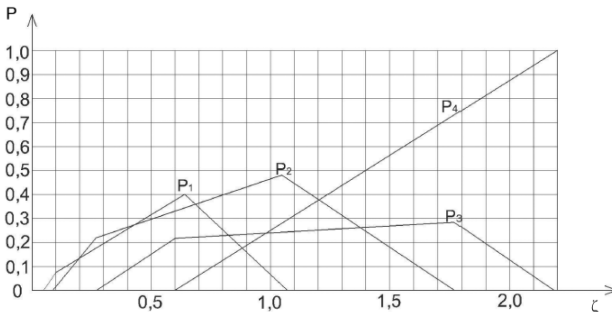
Рисунок 4.1 - Вероятности различной степени разрушения здания (сооружения) и повреждения технологического оборудования в зависимости от величины обобщенного показателя устойчивости, \xi_{\text{зд}}(\xi_{\text{ТО}})
