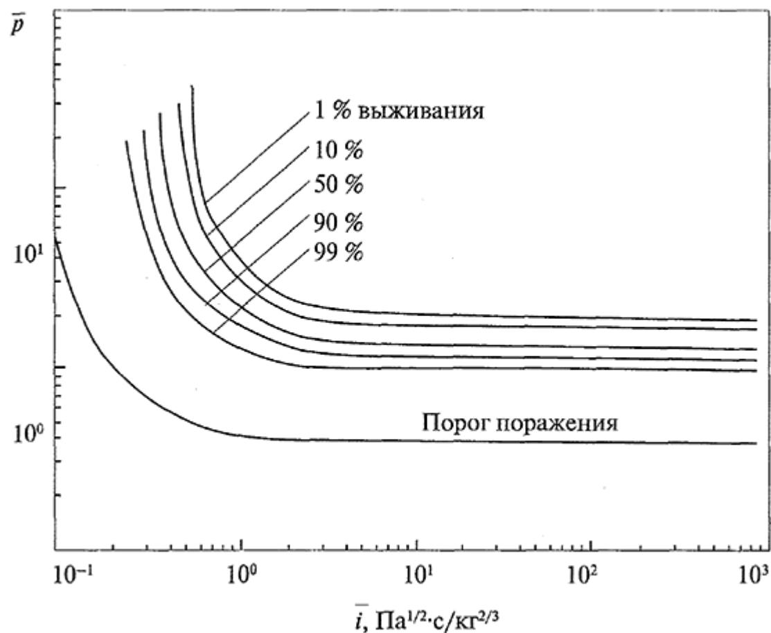
Рисунок 5-3. P - I диаграмма для экспресс-оценки поражения людей от взрыва ТВС при прохождении УВ с отражением (человек находится на открытом пространстве, волна распространяется сверху к земле или человек находится у вертикальной отражающей поверхности, волна распространяется вдоль земли и отражается от вертикальной поверхности)
