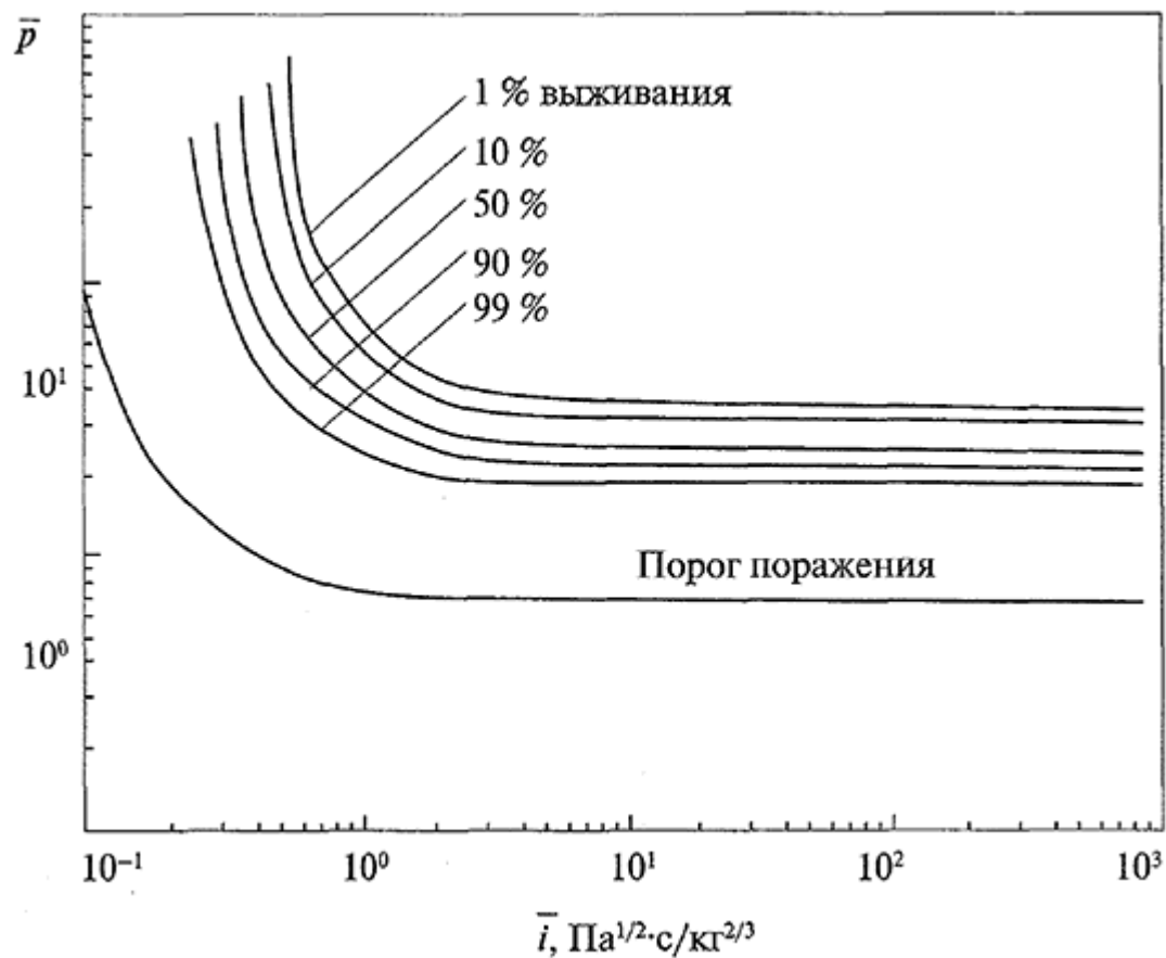
Рисунок 5-2. P - I диаграмма для экспресс-оценки поражения людей от взрыва ТВС при прохождении УВ без ее отражения (человек находится на открытом пространстве, волна распространяется вдоль земли)
