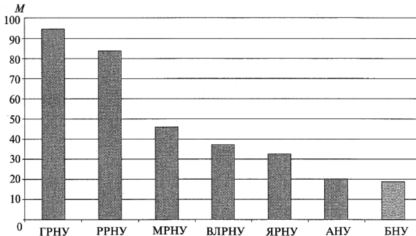
Рисунок 8-4. Ранжирование ОПО по удельным материальным потерям нефти
