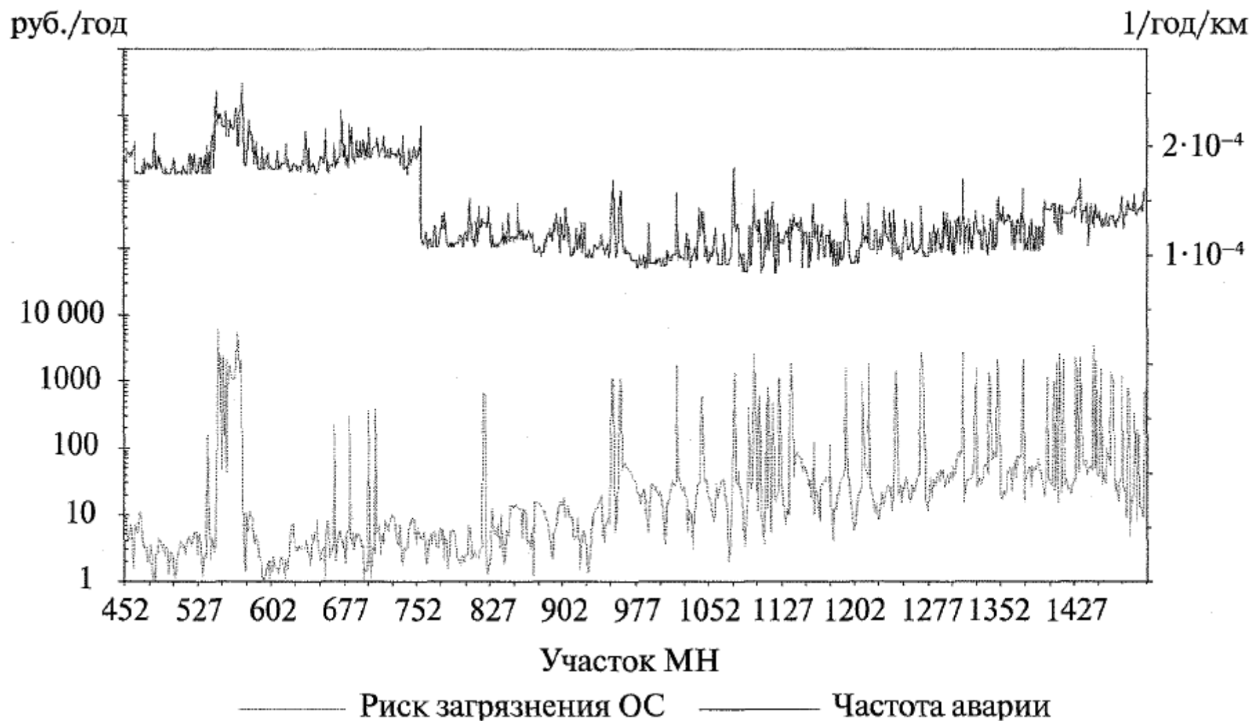
Рисунок 8-3. Пример распределения показателей риска по трассе магистрального нефтепровода (км) и ранжирования ОПО (начало)
