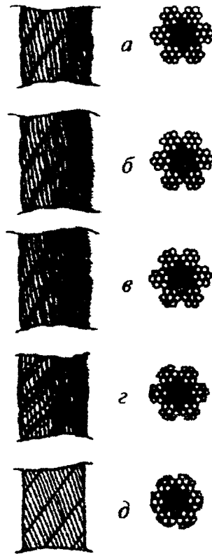
Рисунок 5. Износ наружных проволок каната крестовой свивки: а - небольшие лыски на проводах; б - увеличенная длина лысок на отдельных проволоках; в - удлинение лысок в отдельных проводах при заметном уменьшении диаметра проволок; г - лыски на всех проволоках, уменьшение диаметра каната;
