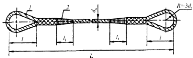
Рис.П.1.25. Универсальный строп, исполнение 1:
