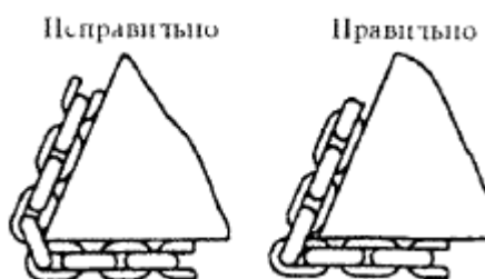
Рис.П.3.2. Строповка грузов цепными стропами
