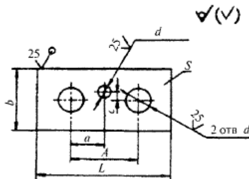
Рис.П.1.5. Планка типа П
