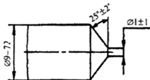
Рис.2. Разделка кромок на концах заготовок из круглого прутка
