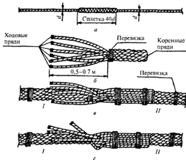
Рис.П.1.20. Сращивание каната
