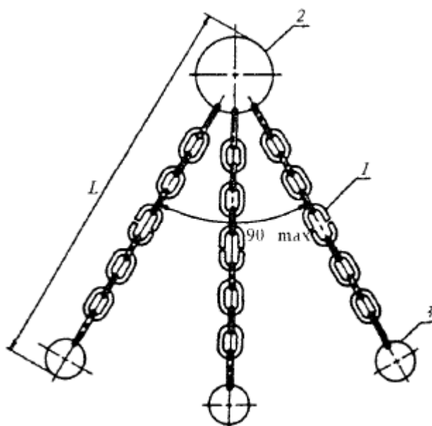
Рис.П.1.29. Трехветвевой строп
