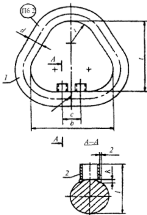
Рис.П.1.8. Звено типа Т, исполнение с двумя упорами
