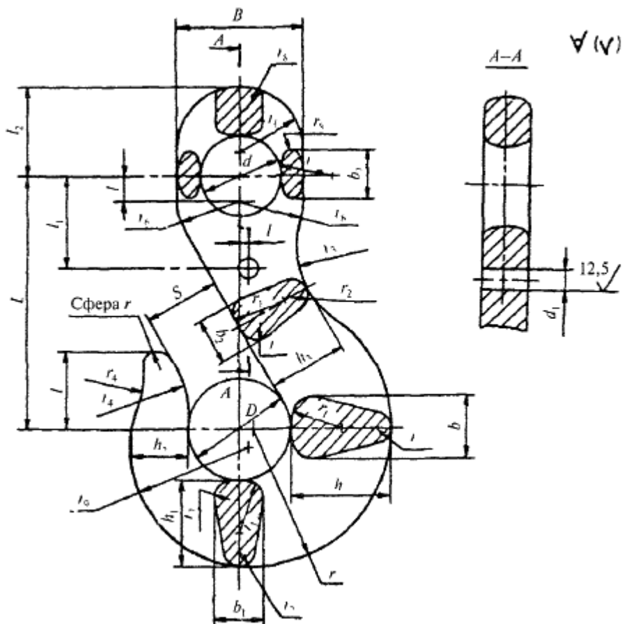
Рис.П.1.13. Крюк стропа
