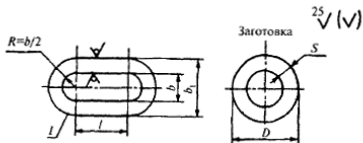
Рис.П.1.19. Втулка
