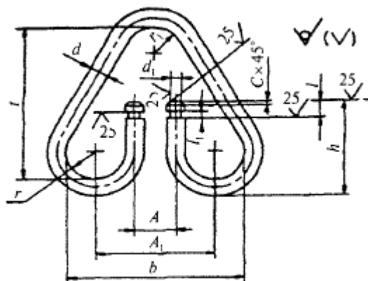
Рис.П.1.3. Скоба типа Ст1
