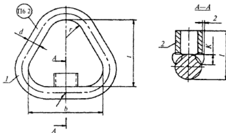
Рис.П.1.6. Звено типа Т, исполнение с одним упором
