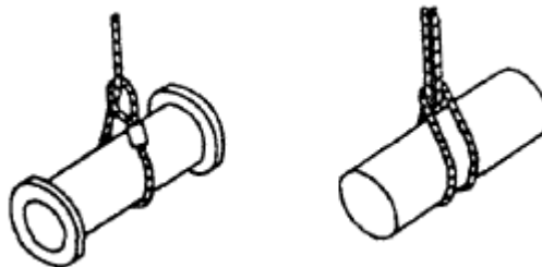
Рис.П.3.4. Стрповка грузов с затяжкой петлей
