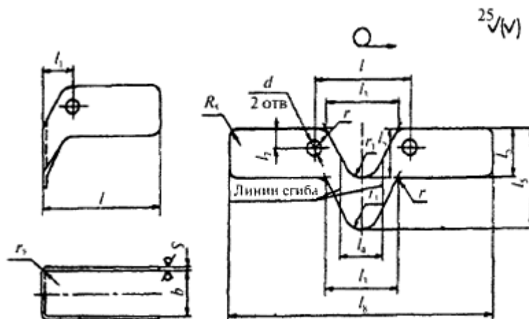
Рис.П.1.14. Замок
