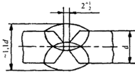
Рис.3. Конструктивные элементы шва сварного соединения
