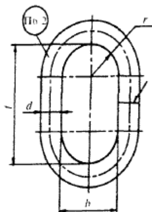
Рис.П.1.11. Звено типа Ов1
