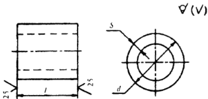
Рис.П.1.9. Упор типа У
