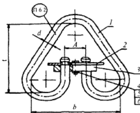
Рис.П.1.2. Звено типа Pt1
