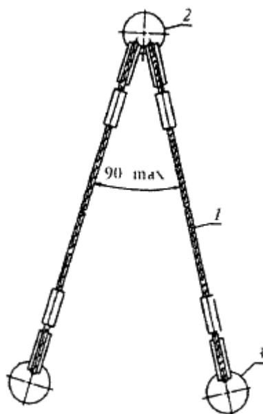
Рис.П.1.22. Двухветвевой строп 1 - канатная ветвь, 2 - звено, 3 - захват
