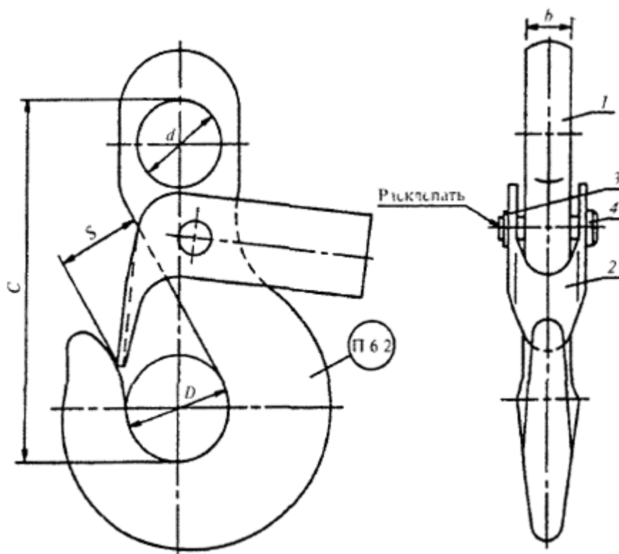
Рис.П.1.12. Крюк типов К1 и К2
