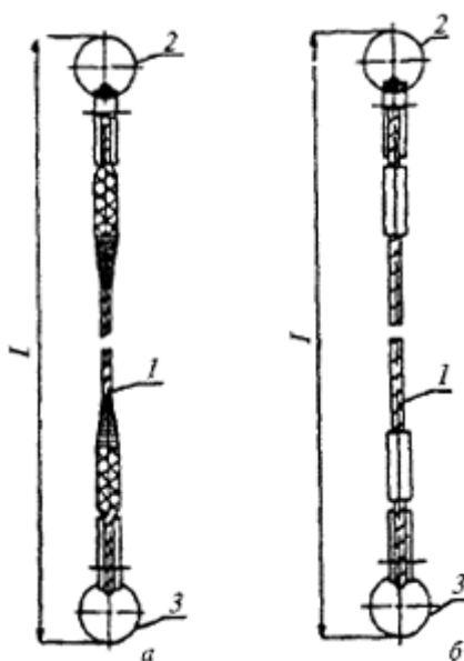
Рис.П.1.21. Одноветвевой строп (заделка концов каната а - заплеткой, б - опрессовкой алюминиевой)
