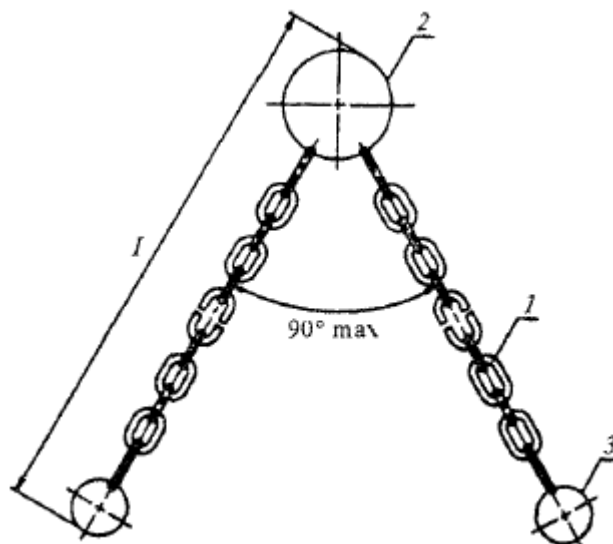
Рис.П.1.28. Двухветвевой строп
