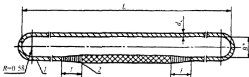
Рис.П.1.26. Универсальный строп, исполнение 2:
