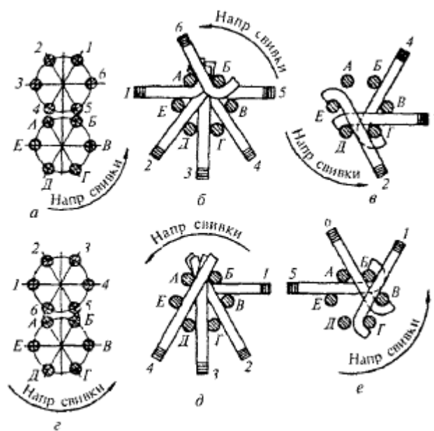
Рис.П.1.16. Схема заплетки каната
