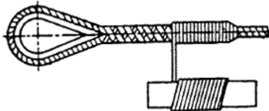
Рис.П.1.17. Изоляция каната
