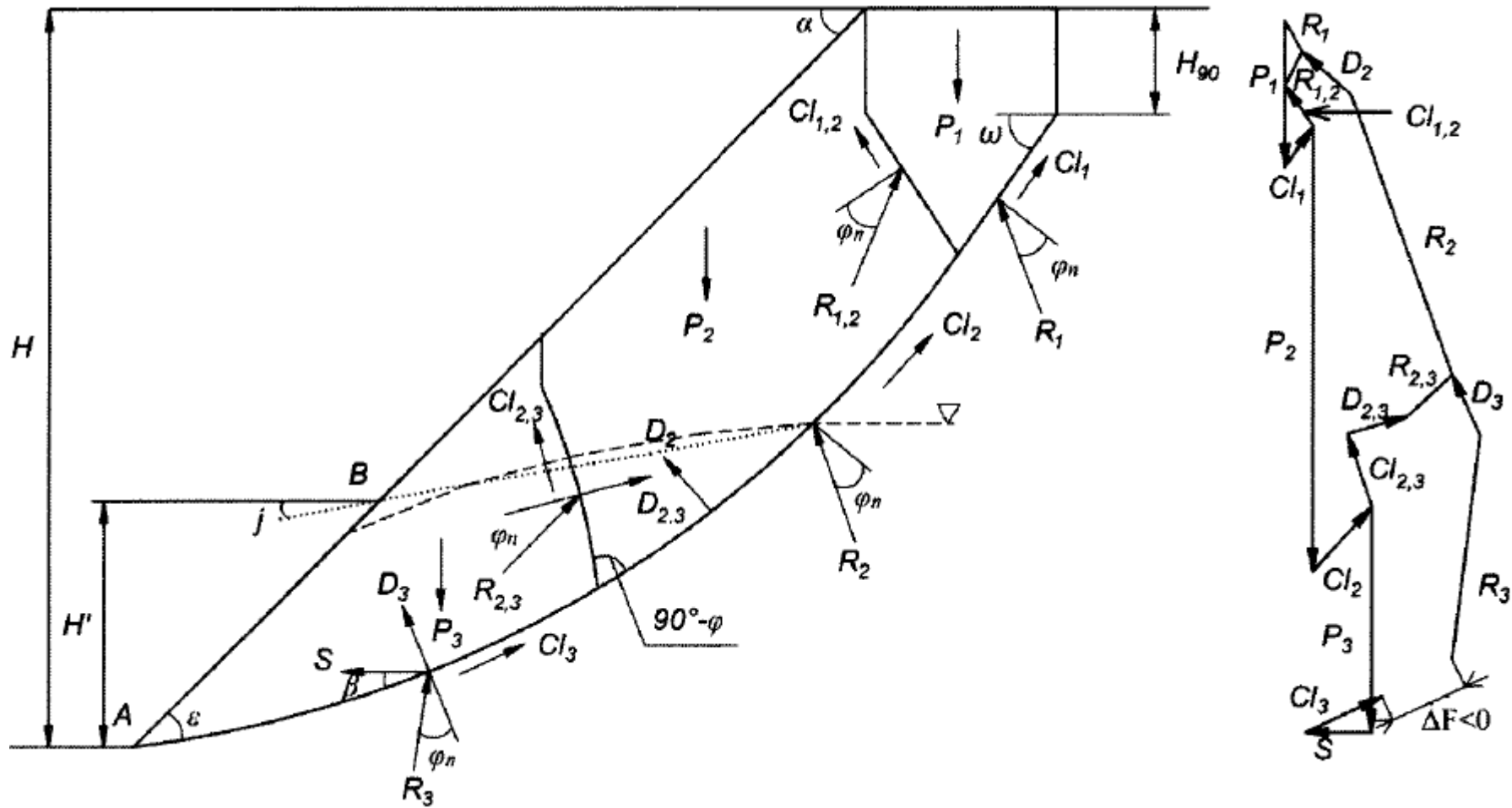
Рисунок 3 - Схема расчёта устойчивости обводнённого изотропного откоса с учётом воздействия сейсмических сил методом векторного сложения сил: P_i - вес рассматриваемого блока, мН; Cl_{i,i+1} , Cl_{i,i-1} , Cl_i - силы сцепления, направленные параллельно соответствующим границам блоков, мН; D_{i,i+1} , D_{i,i-1} , D_i - силы
