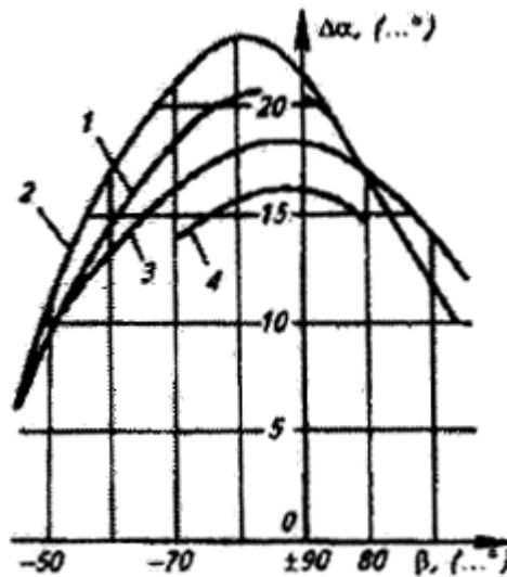
Рисунок 4 - Графики поправок к углам погашения изотропных откосов \alpha_{из} при определении предельных углов наклона бортов в слоистых массивах по схемам 8 и 12 таблицы 2: 1 - \alpha_{из} = 57^\circ, \varphi' = 17^\circ ; 2 - \alpha_{из} = 52^\circ, \varphi' = 17^\circ ; 3 - \alpha_{из} = 52^\circ, \varphi' = 24^\circ ; 4 - \alpha_{из} = 52^\circ, \varphi' = 30^\circ .
