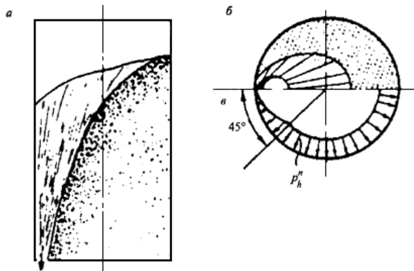
а - разрез силоса; б - план; в - эпюра давления
