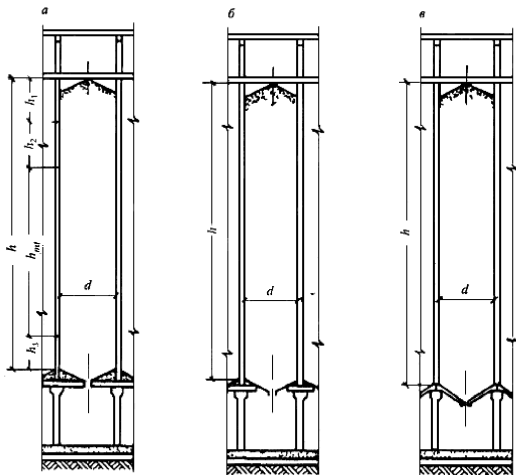
а - с плоским дном и забуткой
