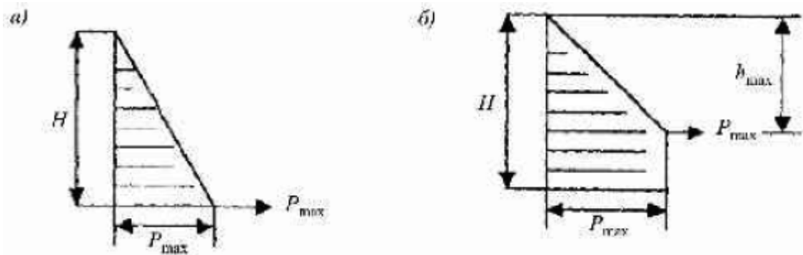
а - гидростатическое давление; б - расчетное давление при уплотнении смеси внутренними вибраторами
