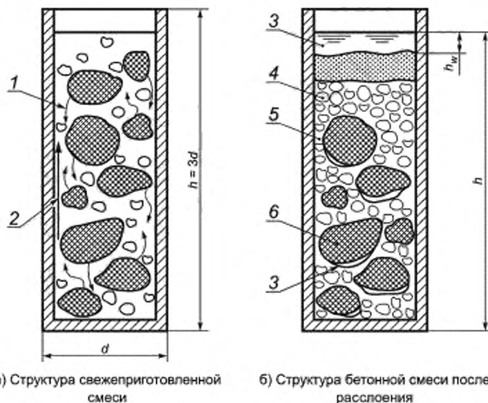
1 — направление движения крупного заполнителя; 2 — направление движения отжимаемой воды; 3 — отделившаяся вода; 4 — цементное тесто; 5 — мелкий заполнитель; 6 — крупный заполнитель
