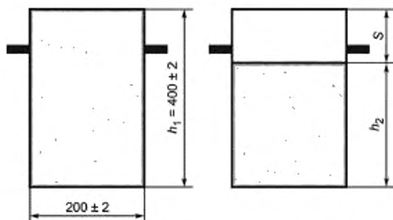
Рисунок 5 — Расчетная схема степени уплотняемости (бетонная смесь в форме до и после уплотнения)
