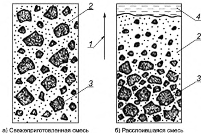
Рисунок 8 — Расслоение бетонной смеси при длительных вибрационных воздействиях
