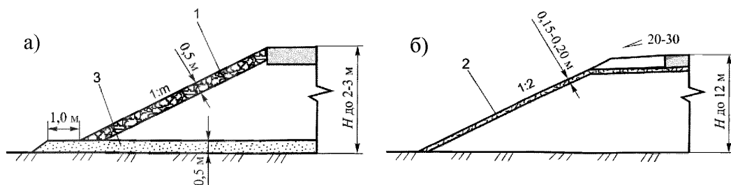
Рисунок 62 – Основные конструктивные решения конструкций с изолирующими слоями для откосов насыпей в зоне подвижных песков
