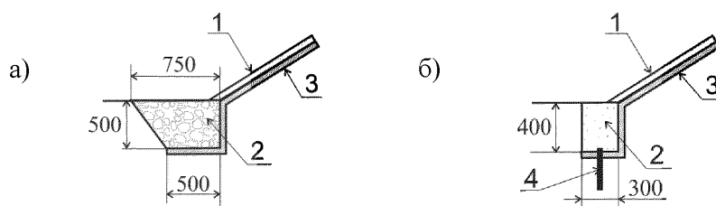
1 – растительный грунт с посевом трав; 2 – призма из гравийных, щебеночных или песчаных материалов; 3 – геосинтетический материал; 4 – анкер
