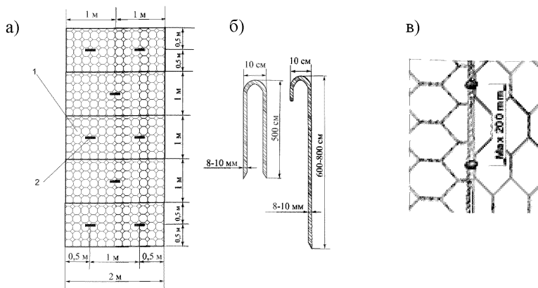
1 – матрацно-тюфячные габионные конструкции; 2 – анкер
