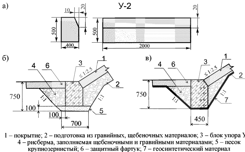
Рисунок 55 – Схемы конструктивного решения упорной конструкции с применением унифицированного бетонного блока У-2: для подтопляемых откосов при наличии размывов (а); с применением традиционных строительных материалов (б); с применением геосинтетических материалов (в)
