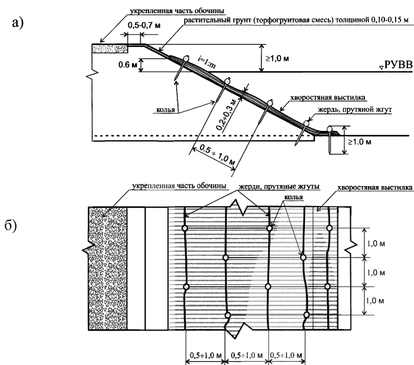
Рисунок 11 – Защитная конструкция укрепления откосов биологического типа при укреплении хворостяной выстилкой: схема конструктивного решения (а); схема расположения по откосу в плане (б)
