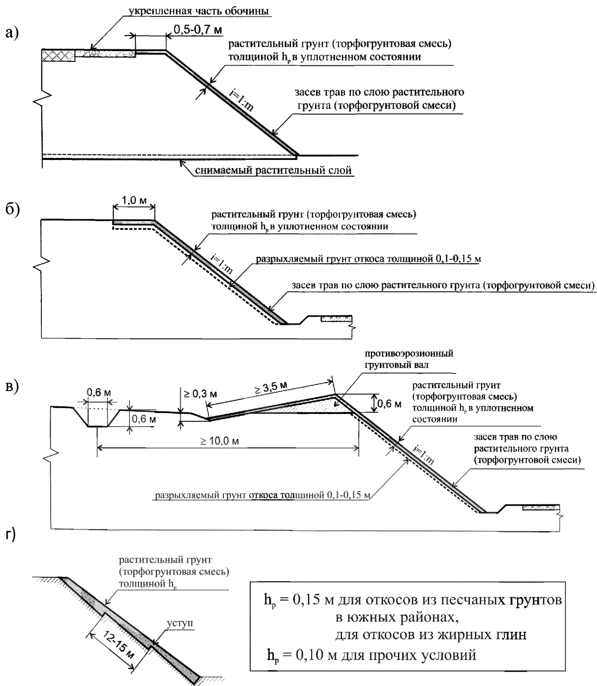
Рисунок 4 – Защитная конструкция укрепления откосов биологического типа (подтип I-1) выполненная методами механизированного посева трав по слою растительного грунта или торфопесчаной смеси: в насыпи (а); в выемке (б); в выемке с устройством противозерозионного вала (банкета) и забанкетной канавы (в); с нарезкой уступов в грунте откоса при длине откоса более 12 м
