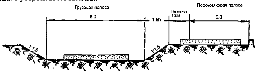
Рисунок 10.11 – Поперечный профиль двухпутного зимника с устройством выемки
