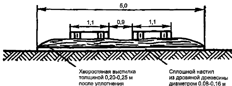
Рисунок 10.3 – Поперечный профиль лесных дорог из деревянных щитов на болотах типа II с толщиной торфа до 2 м
