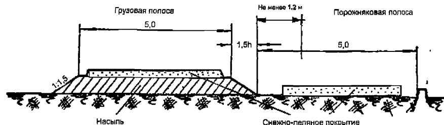
Рисунок 10.10 – Поперечный профиль двухпутного зимника с устройством насыпи
