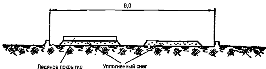
Рисунок 10.9 – Двухпутный зимник в нулевых отметках
