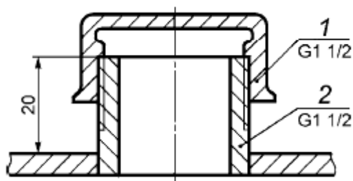
1 - крышка; 2 - газовая труба
