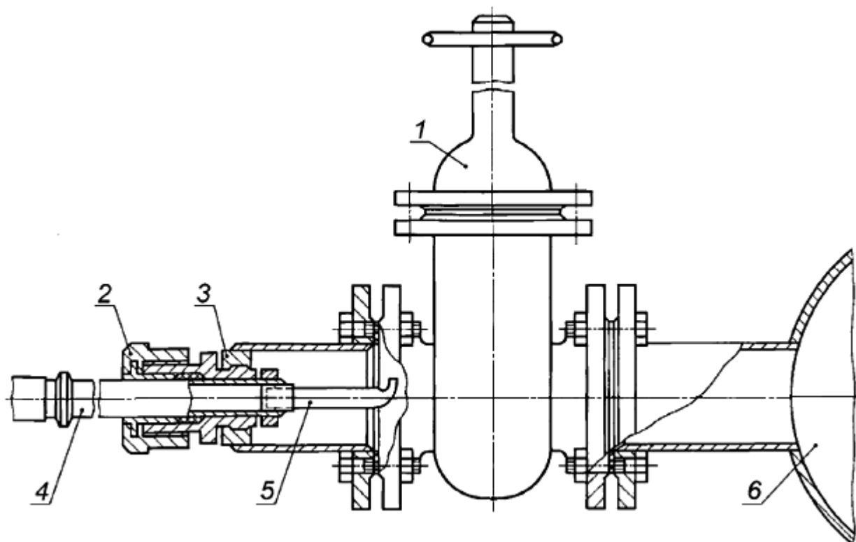
Рисунок В.1 - Шлюзовый затвор для отбора проб под давлением
