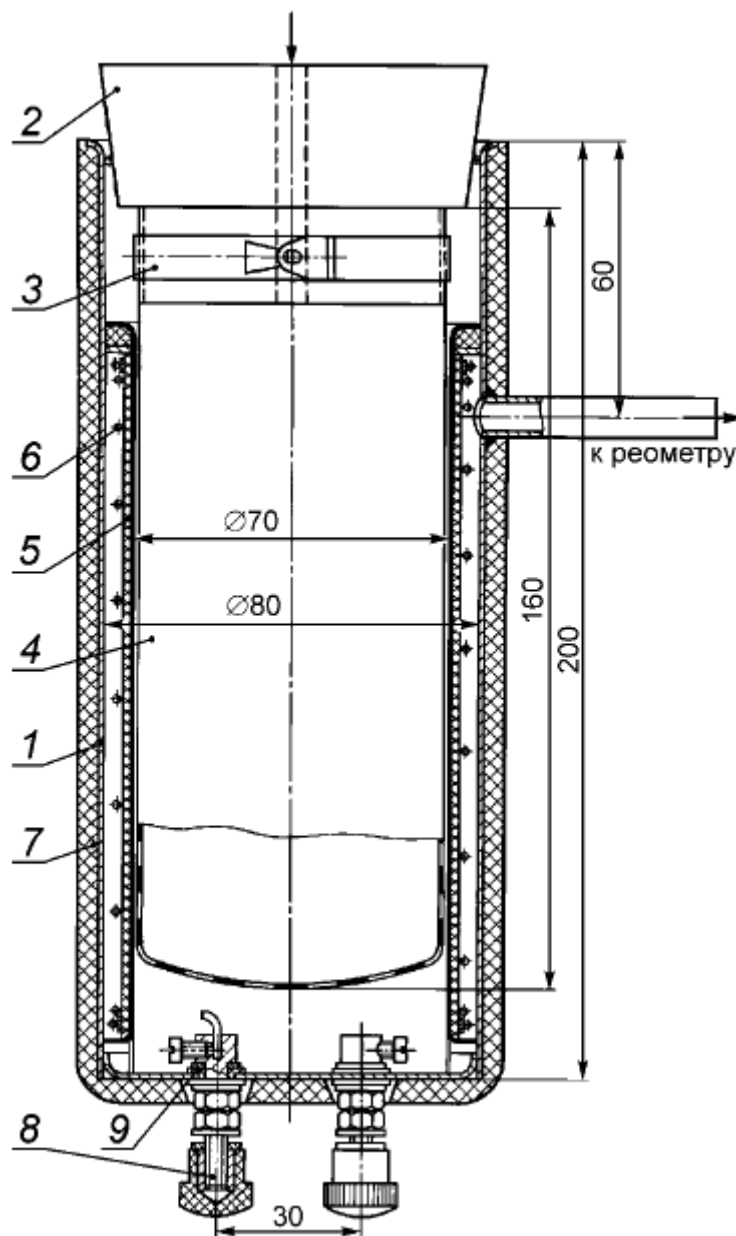
1 - корпус; 2 - резиновая пробка; 3 - хомут; 4 - фильтровальный мешок; 5 - стакан; 6 - электрообогрев; 7 - тепловая изоляция; 8 - контакты; 9 - текстолитовая втулка
