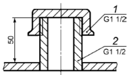
1 - крышка; 2 - газовая труба
