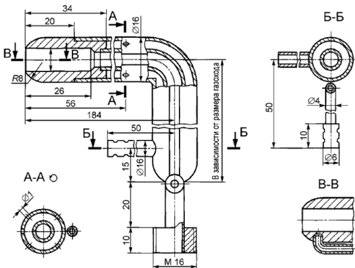
Рисунок А.3 - Пылезаборная трубка нулевого типа
