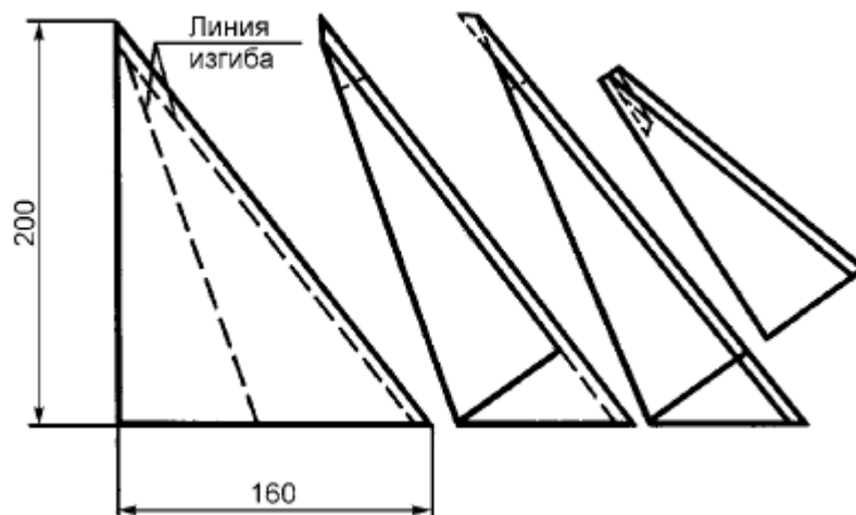
Рисунок Д.3 - Раскрой бумажного фильтра
