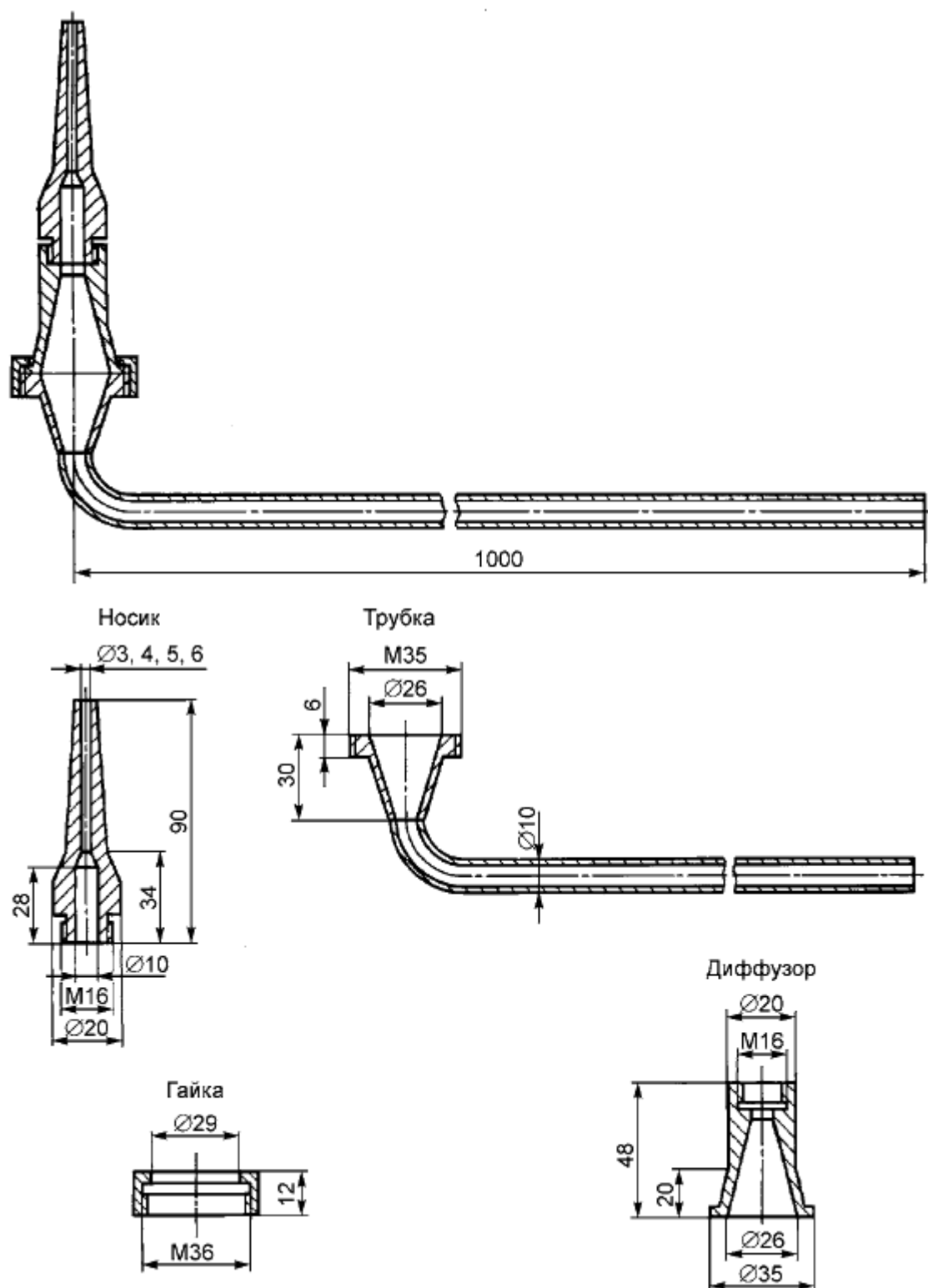
Рисунок Г.3 - Держатель мембранных фильтров АФА
