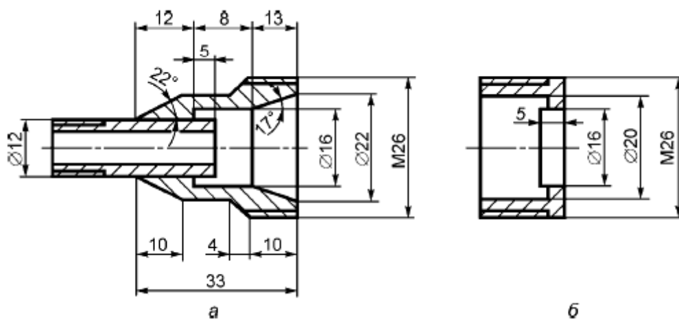
Рисунок Г.1 - Фильтровальные патроны
