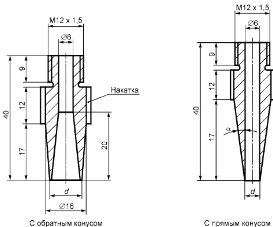
Рисунок А.2 - Наконечники для пылезаборных трубок
