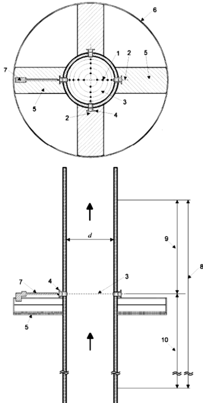
1 - измерительная точка; 2 - измерительная линия; 3 - измерительная плоскость; 4 - измерительный порт; 5 - свободная зона; 6 - место измерений; 7 - линия для ручного отбора проб; 8 - измерительная секция; 9 - участок трубы после измерительной плоскости; 10 - участок трубы до измерительной плоскости
