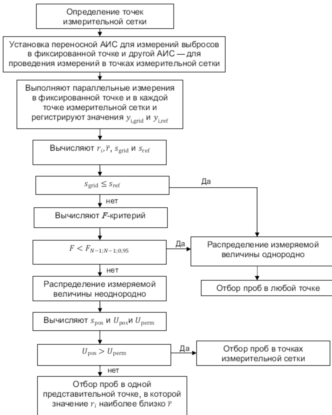
Рисунок 5 - Схема методики определения однородности
