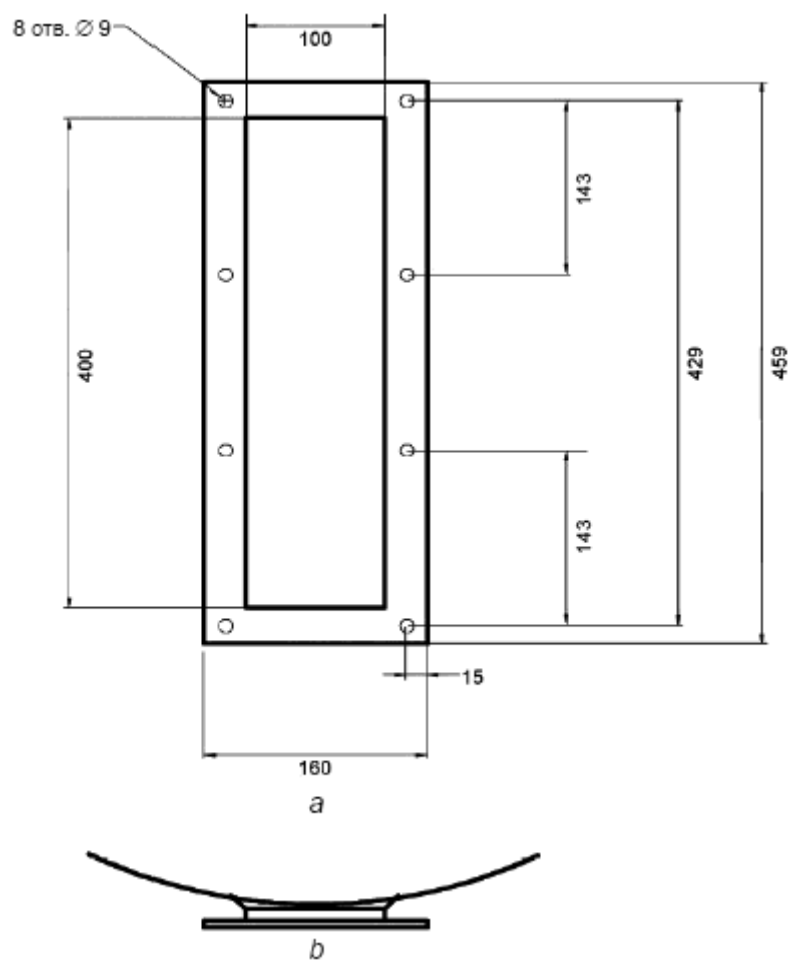
Рисунок А.1 - Пример прямоугольного измерительного порта
