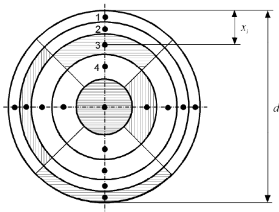
Рисунок D.1 - Размещение точек отбора проб в круглых газоходах с диаметром более 2 м в соответствии с общим правилом
