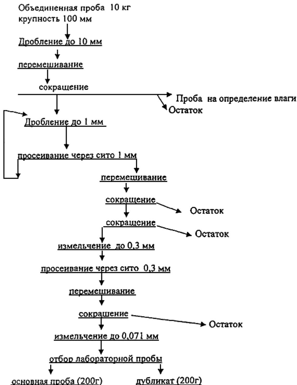
Рис.1. Примерная схема подготовки лабораторной пробы
